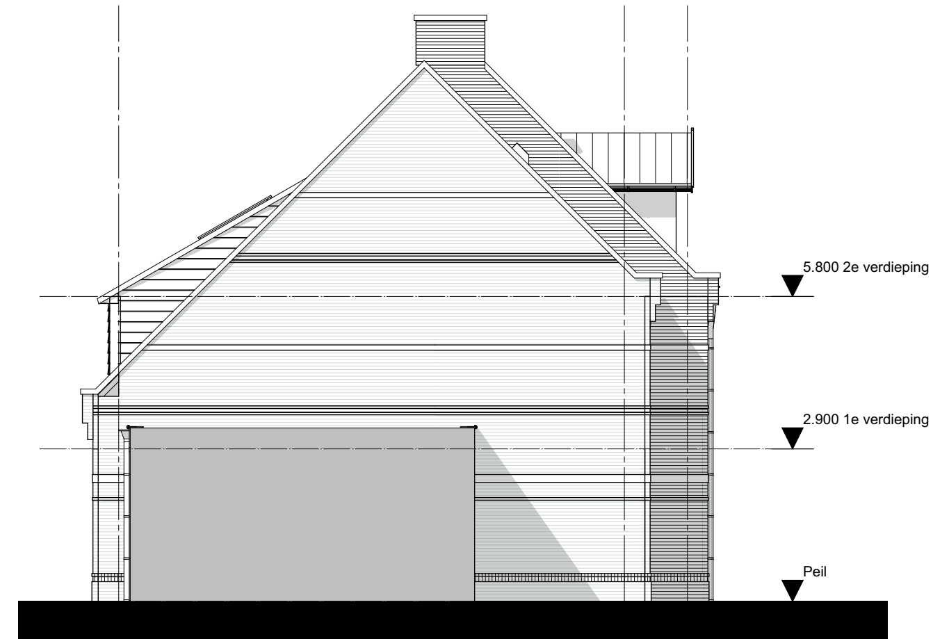
Linkergevel
