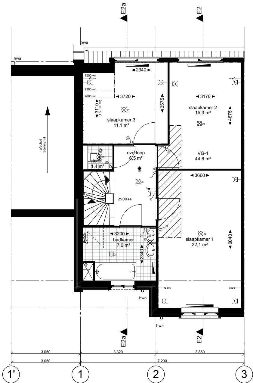
1e verdieping 1:100
