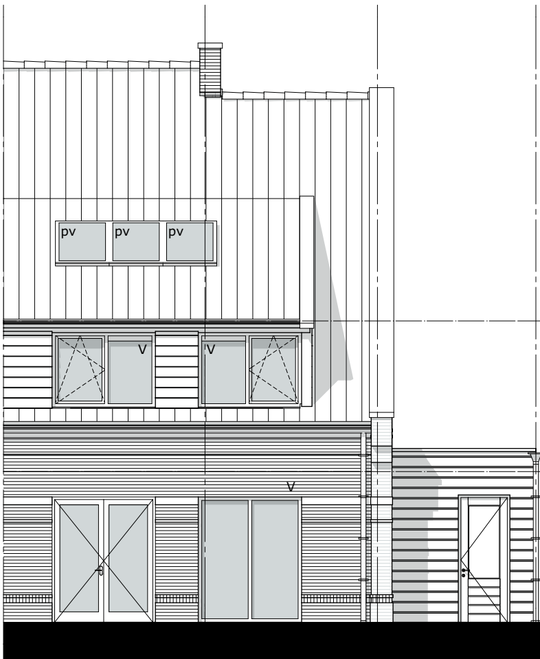
Achtergevel 1:100
