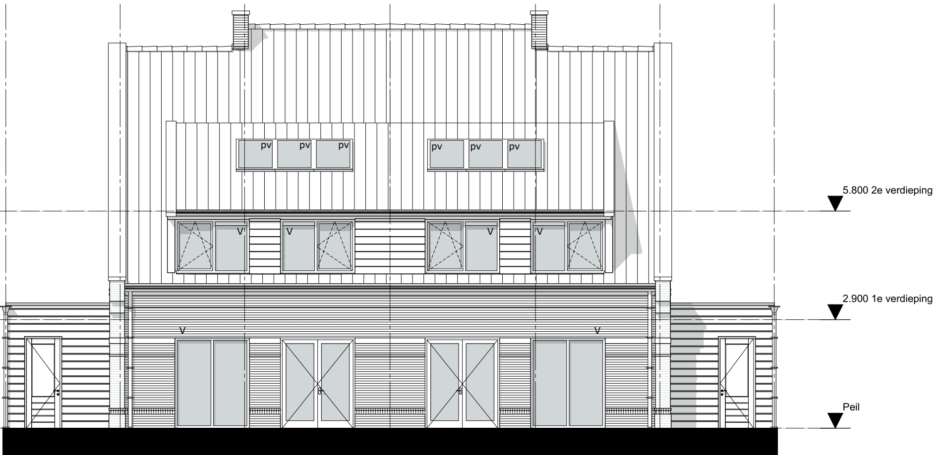
Achtergevel
