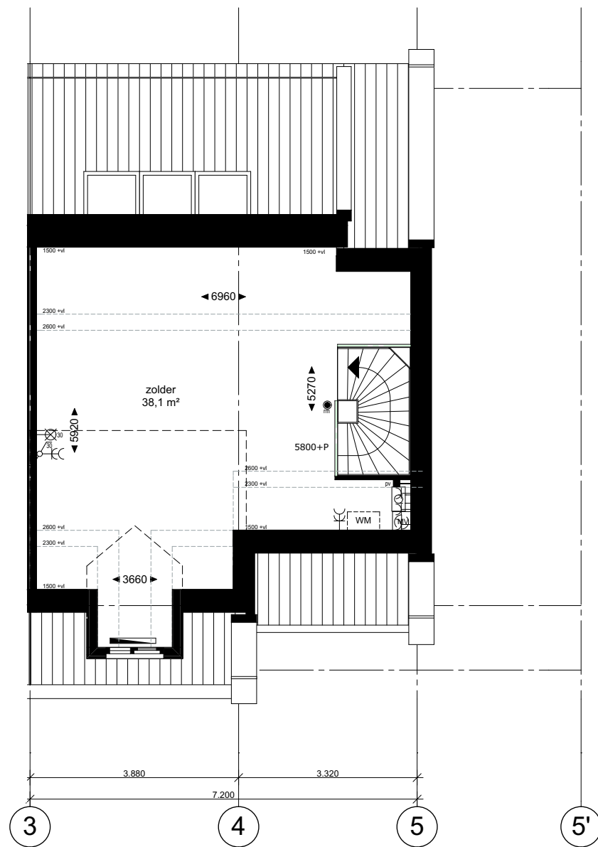
2e verdieping 1:100
