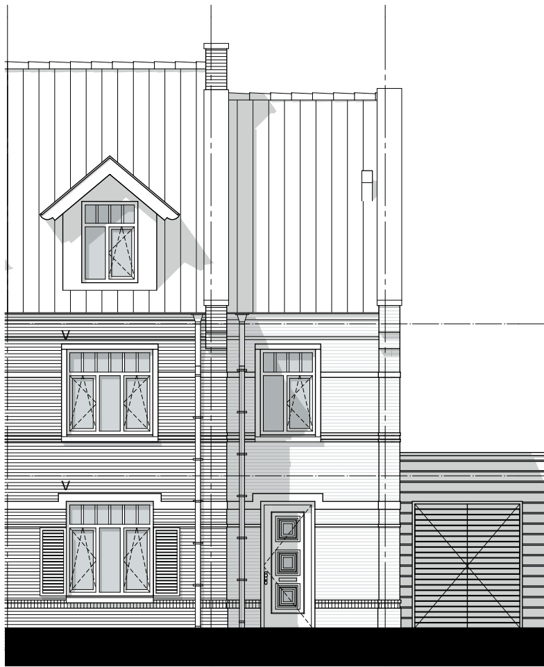
Voorgevel 1:100
