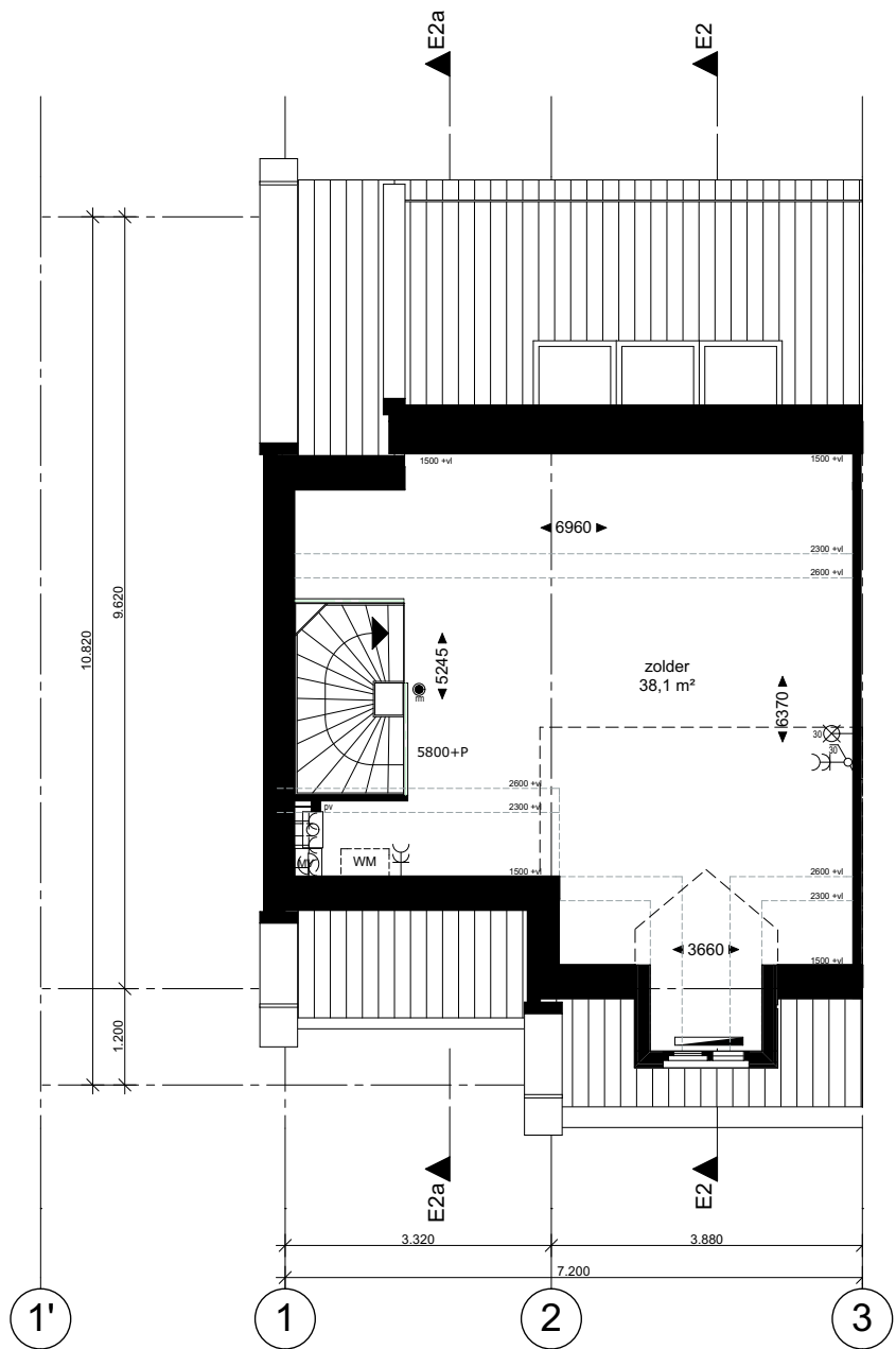
2e verdieping 1:100
