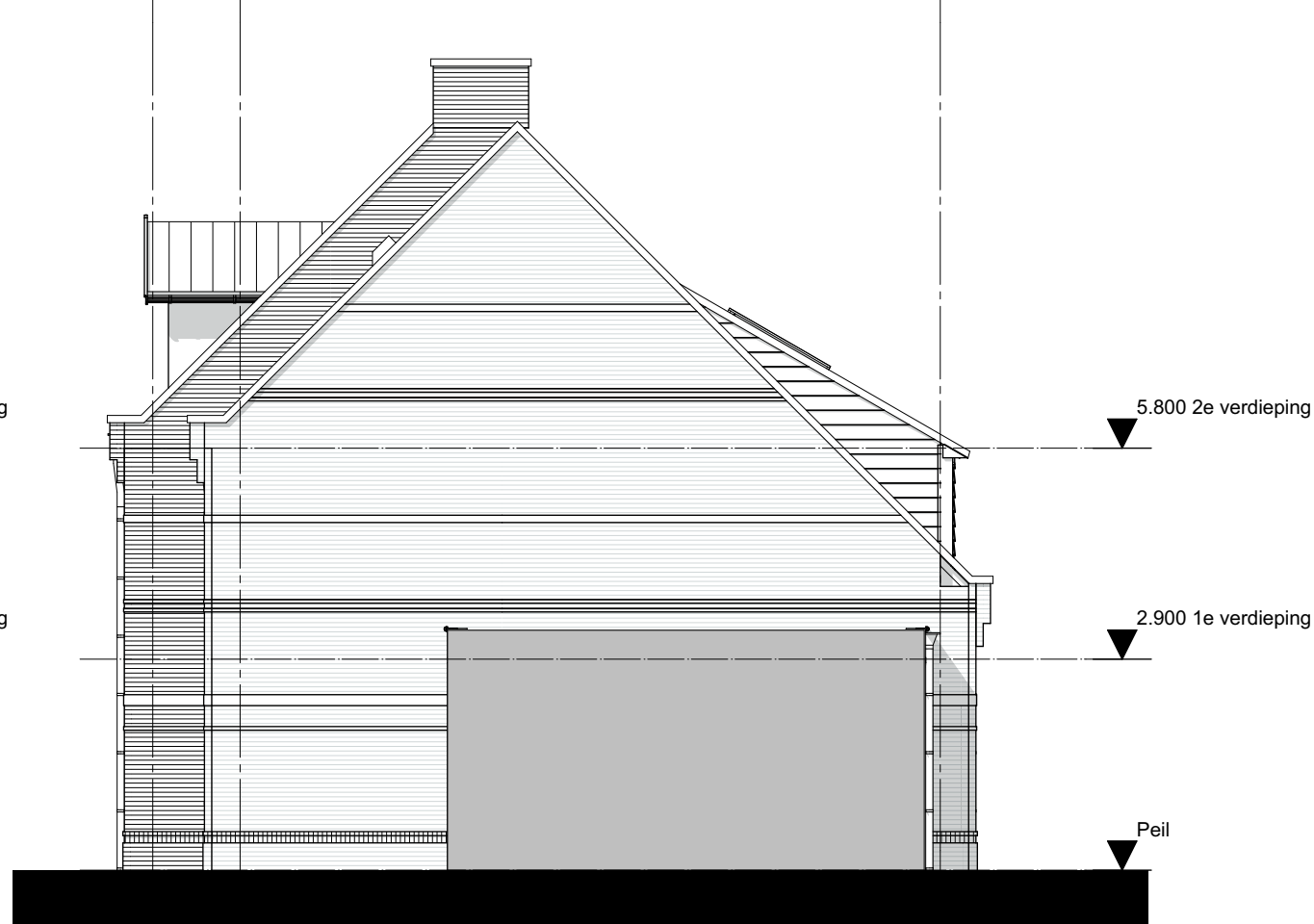
Rechtergevel
