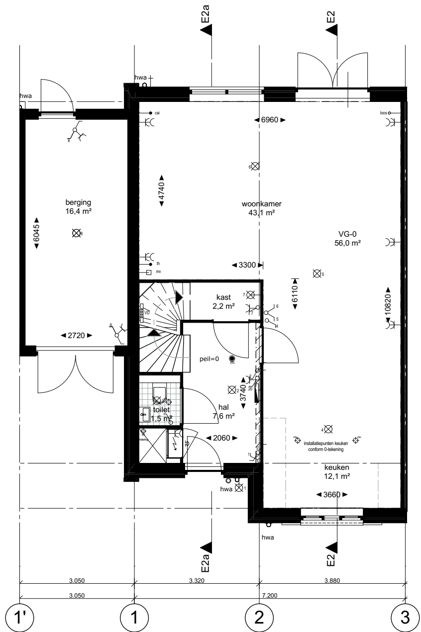
Begane grond 1:100
