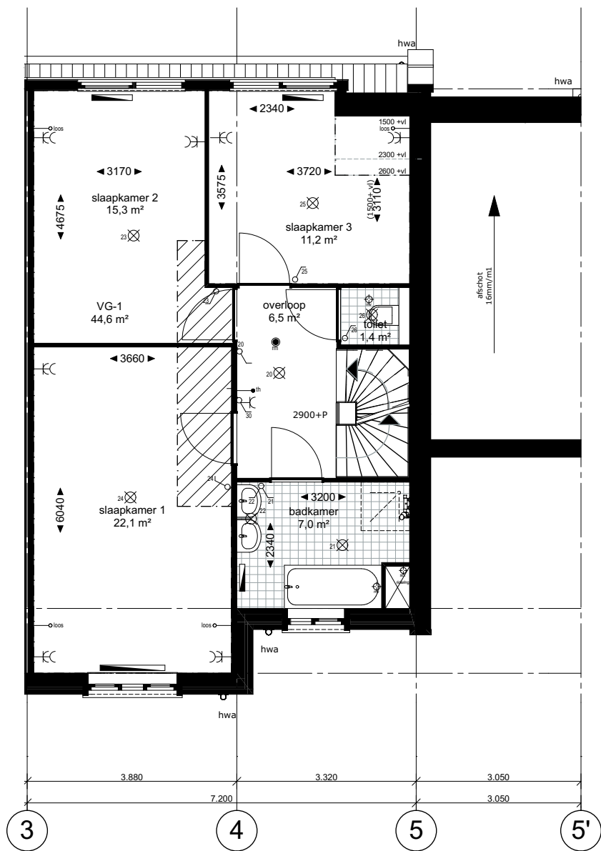
1e verdieping 1:100
