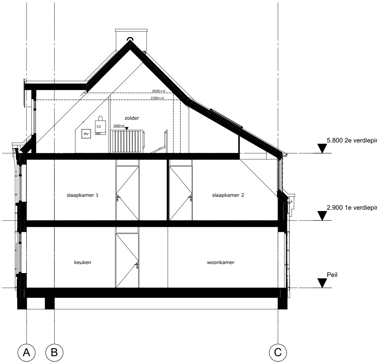
Doorsnede E2-E2 1:100
