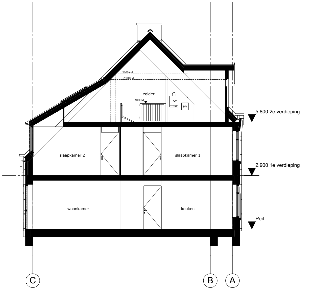
Doorsnede E2-E2 1:100
