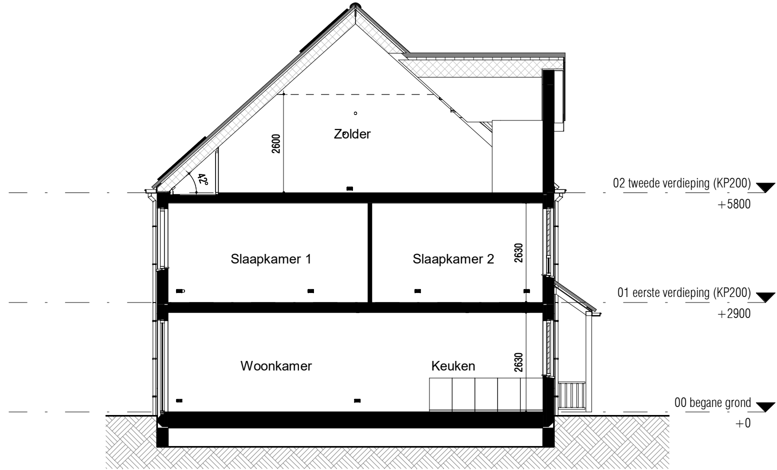
Doorsnede (1:100)
