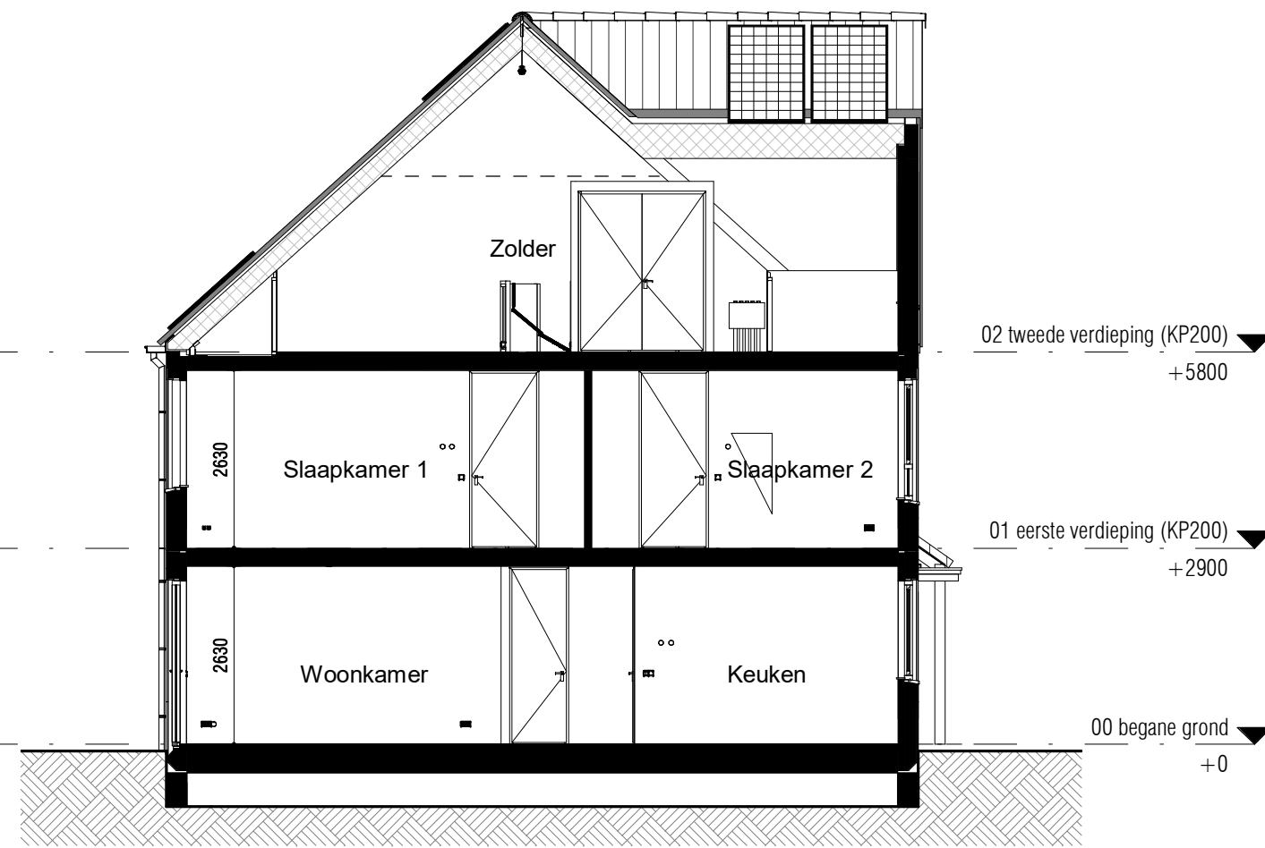
Doorsnede (1:100)
