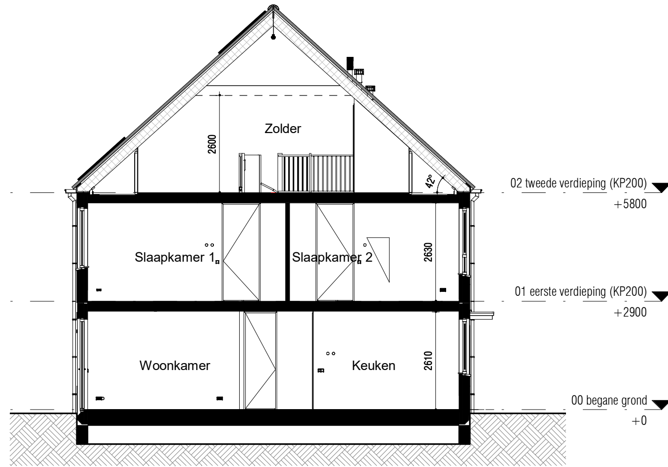
Doorsnede (1:100)
