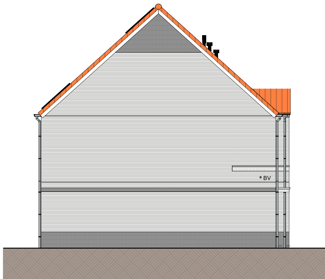
Linkerzijaanzicht (1:100)
