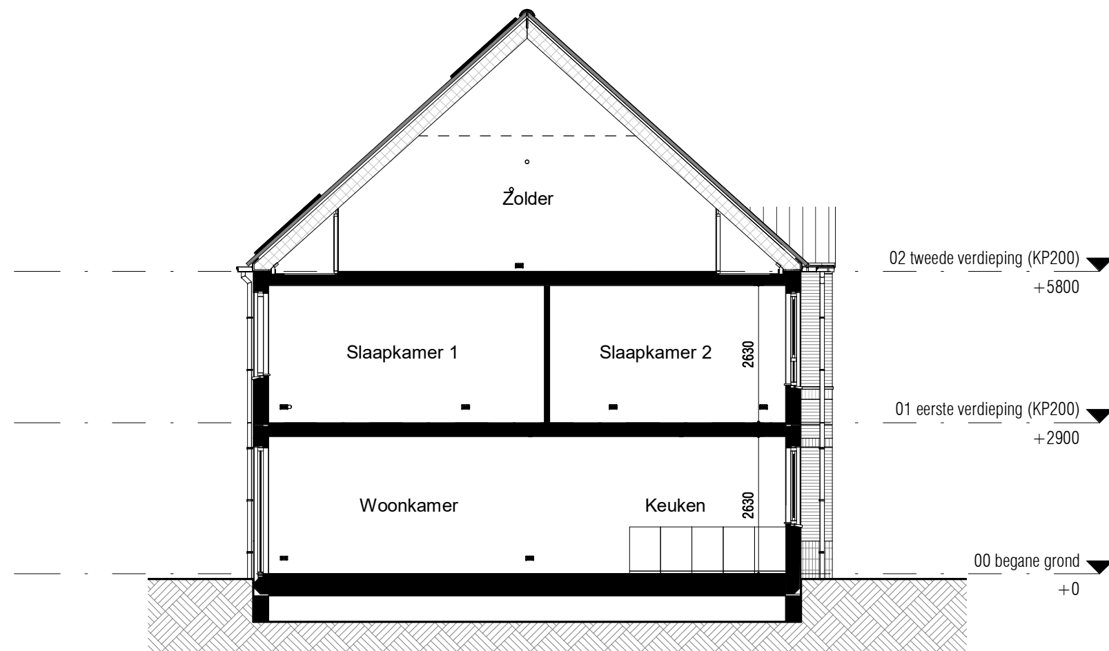
Doorsnede (1:100)
