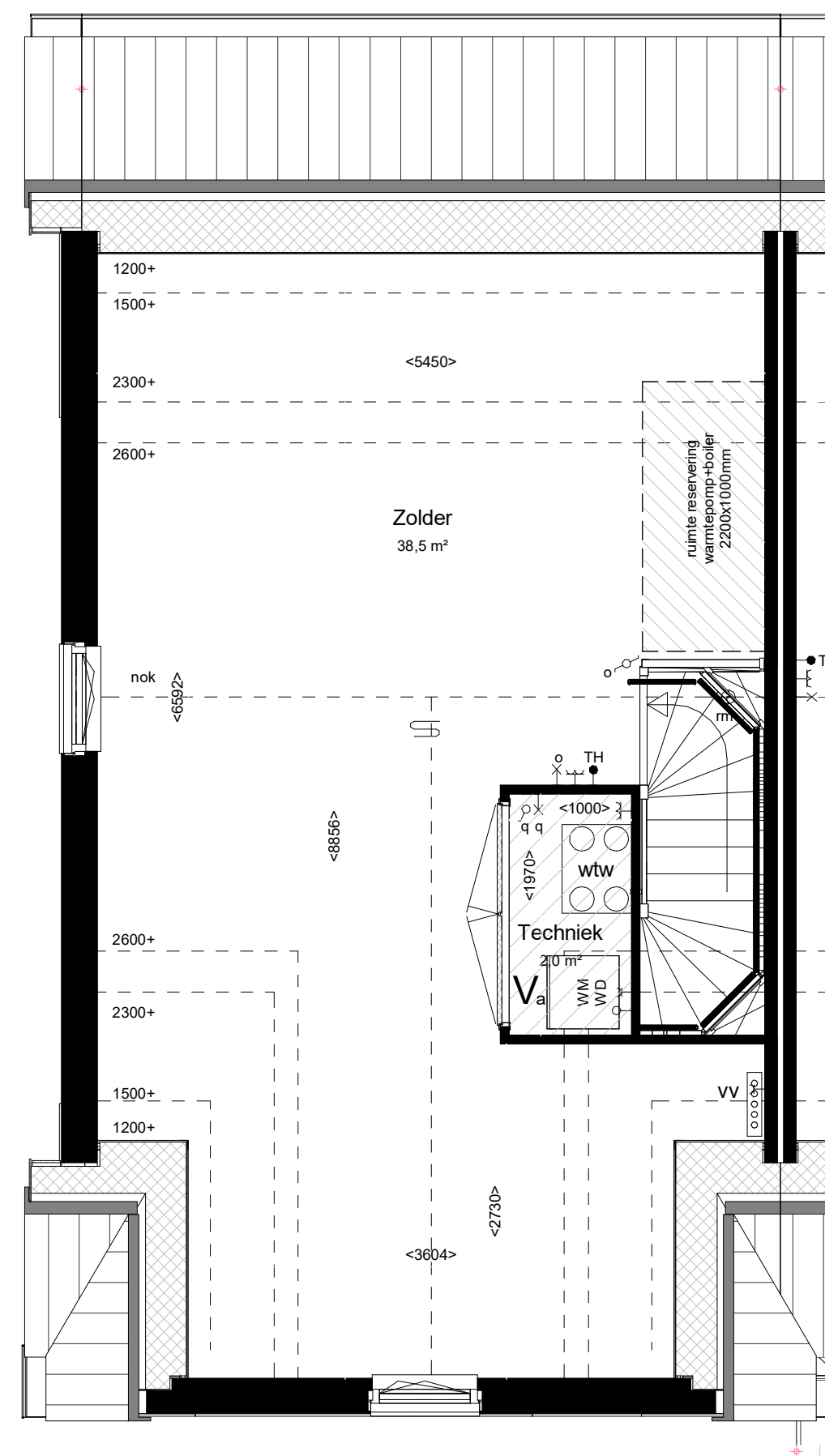
Tweede verdieping 5800+P
