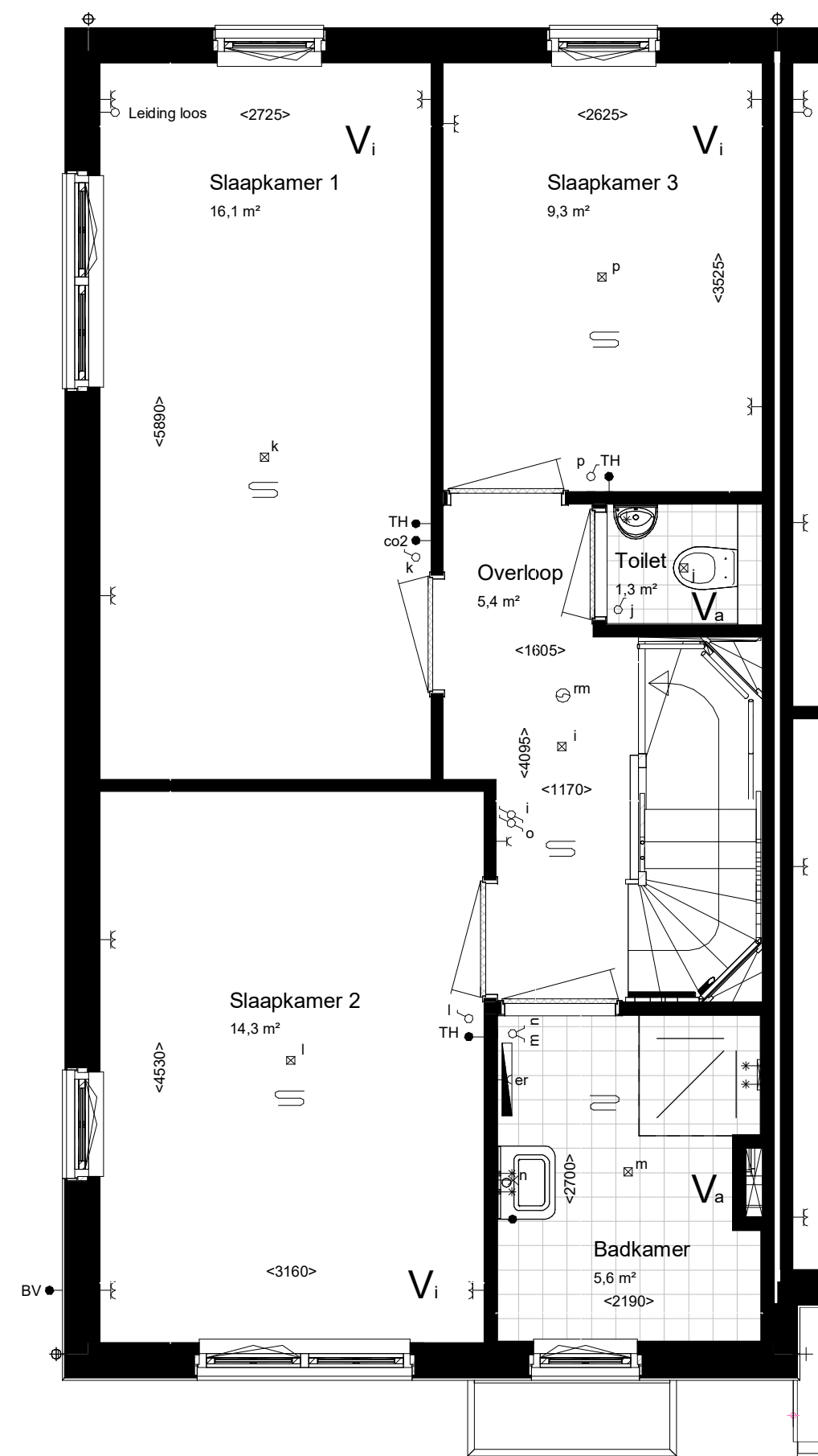
Eerste verdieping 2900+P
