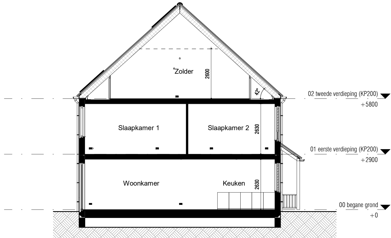
Doorsnede (1:100)
