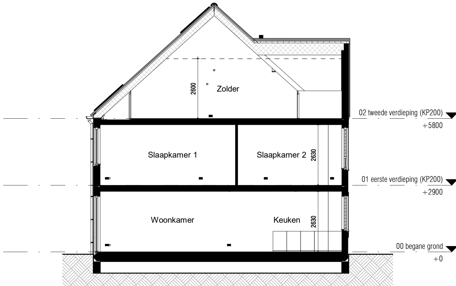
Doorsnede (1:100)
