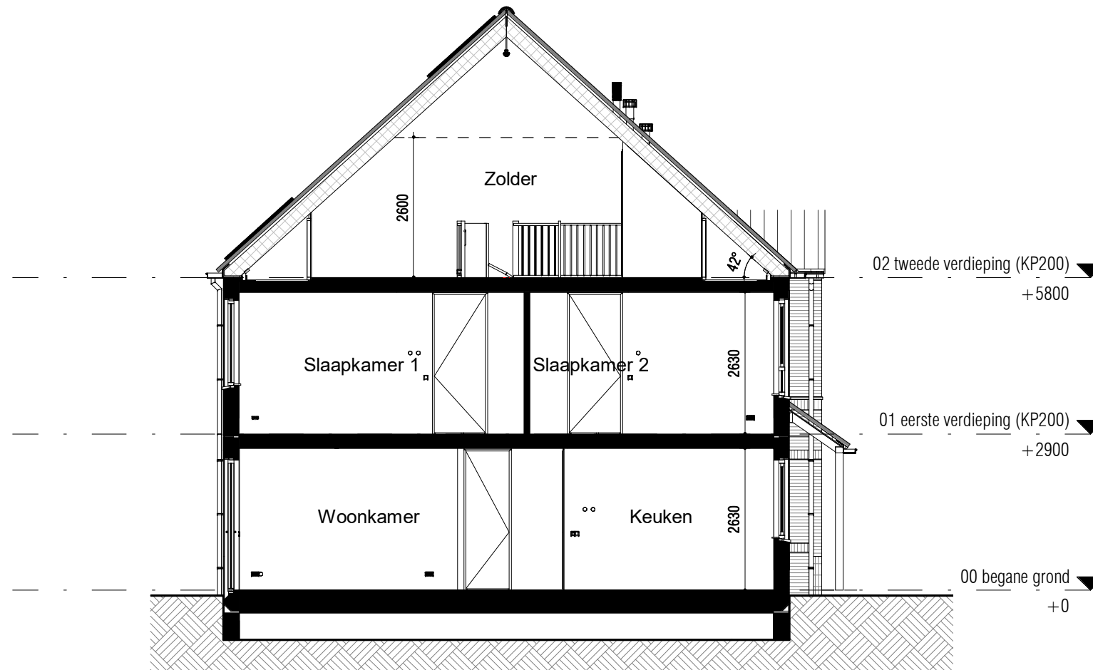
Doorsnede A
