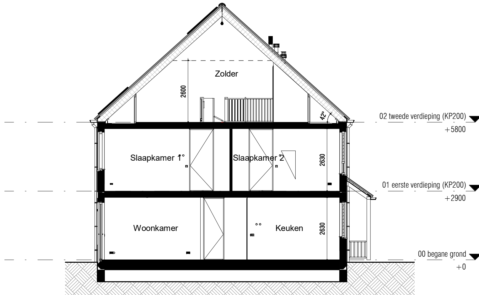
Doorsnede (1:100)
