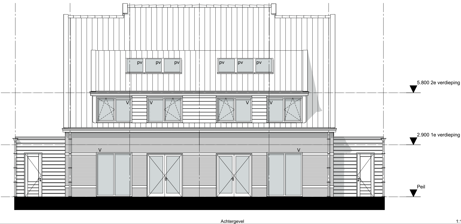
Achtergevel
