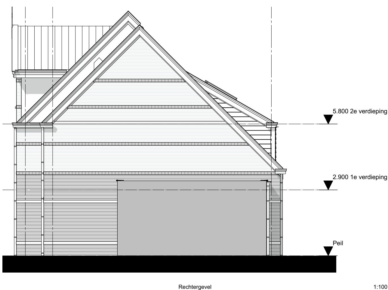
Rechtergevel
