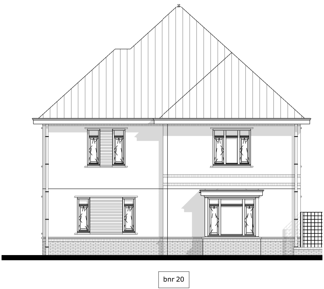
rechter gevel
