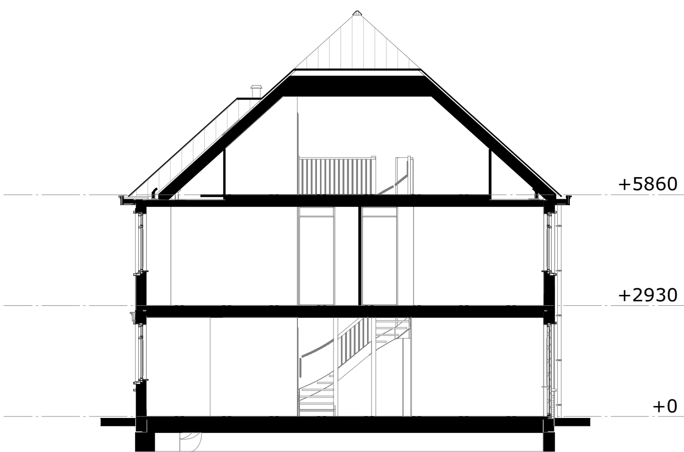
doorsnede A
