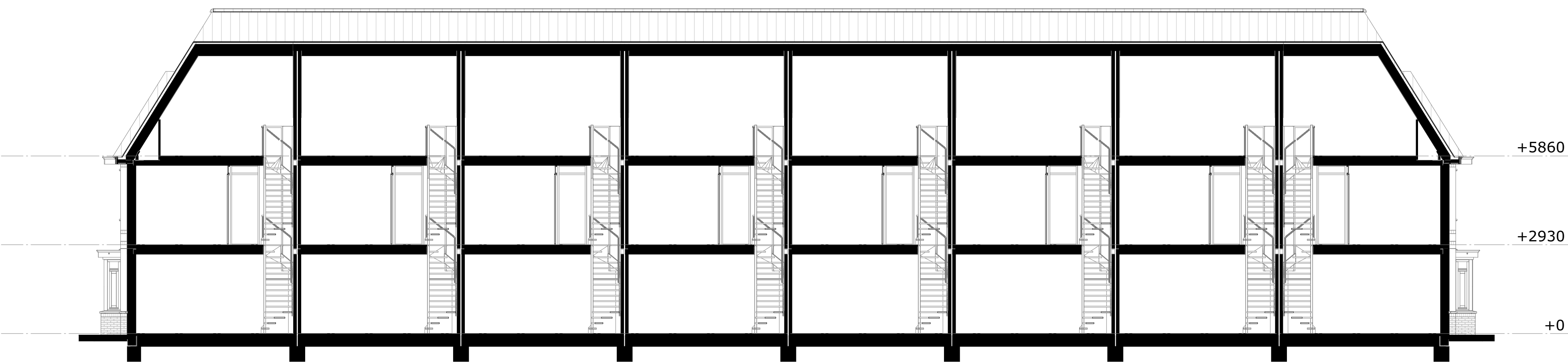
doorsnede B
