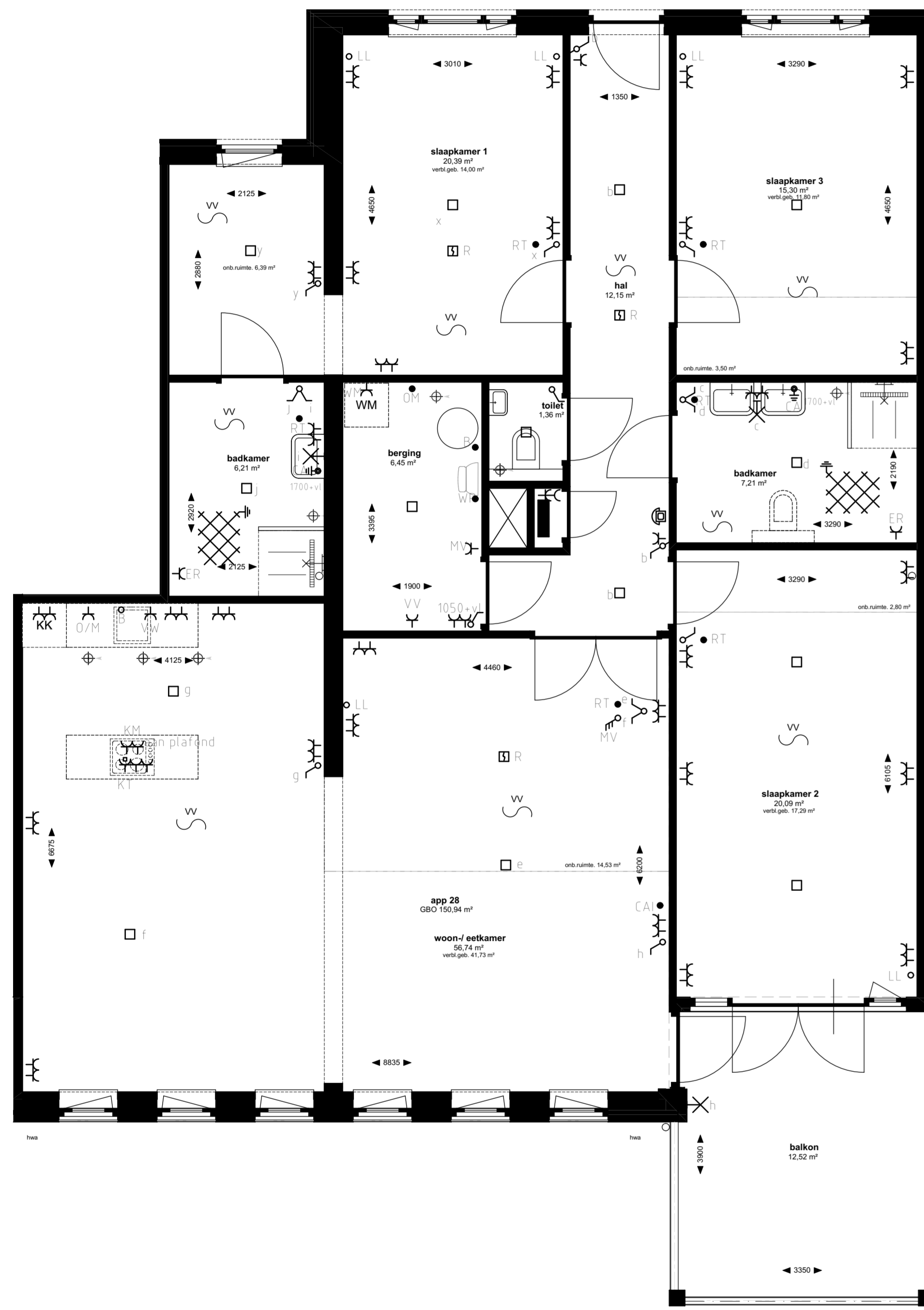
Appartement 28 (1:50)
