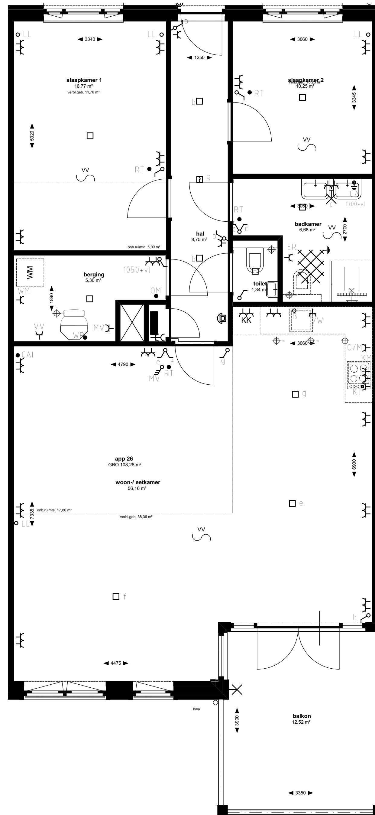
Appartement 26 (1:50)
