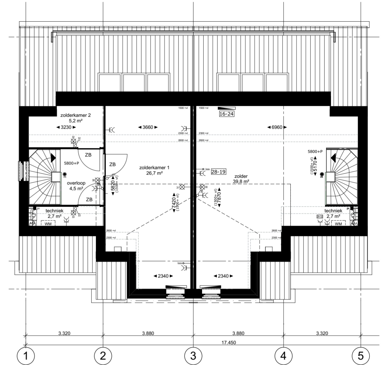
2e verdieping 1:100
