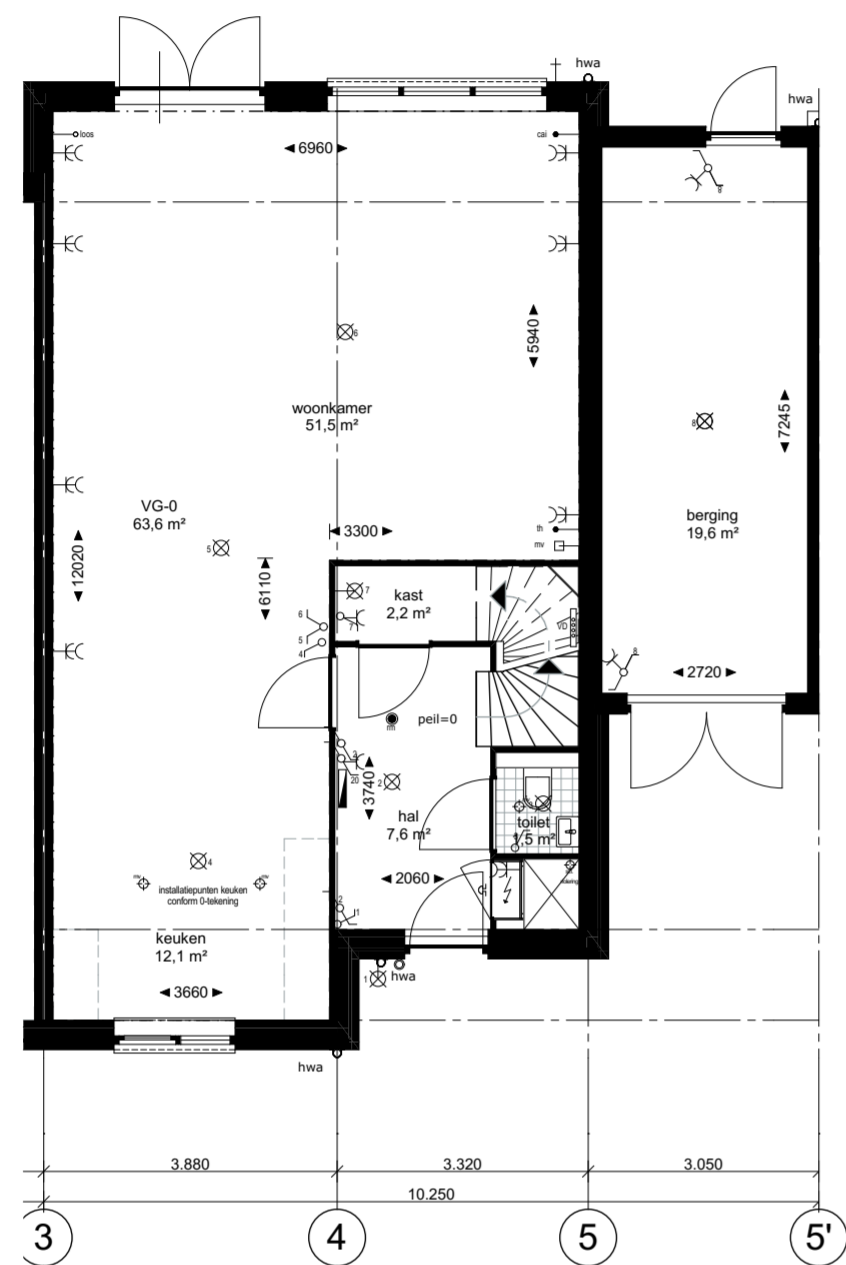
Begane grond 1:100
