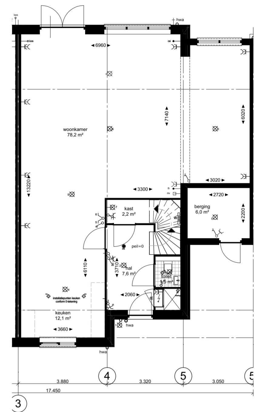
Begane grond 1:100
