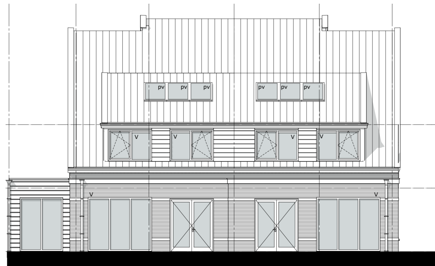
Achtergevel 1:100
