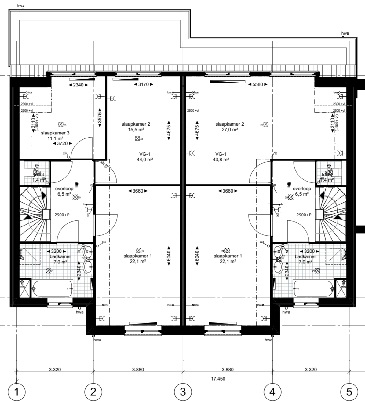
1e verdieping 1:100
