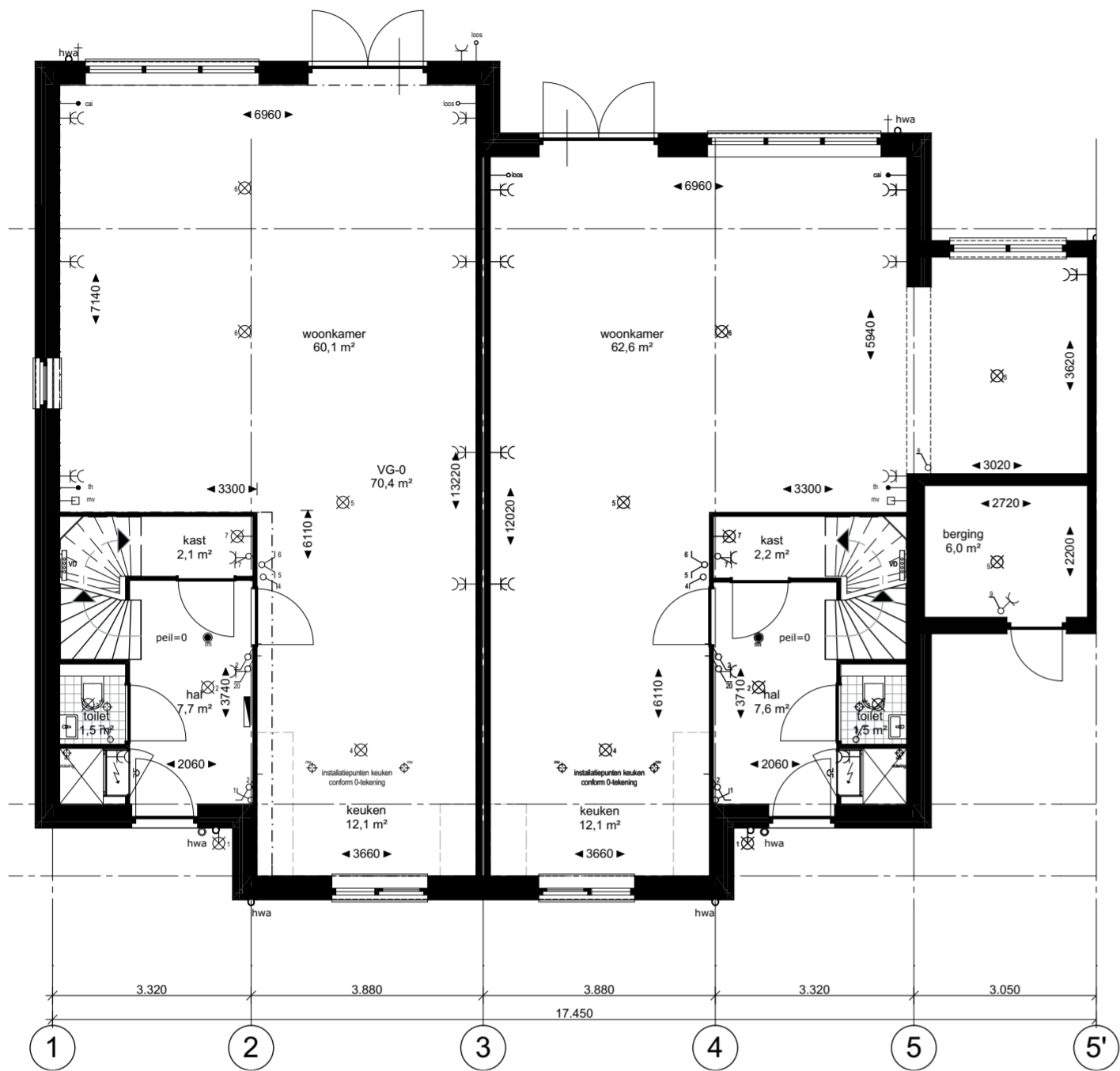
Begane grond 1:100
