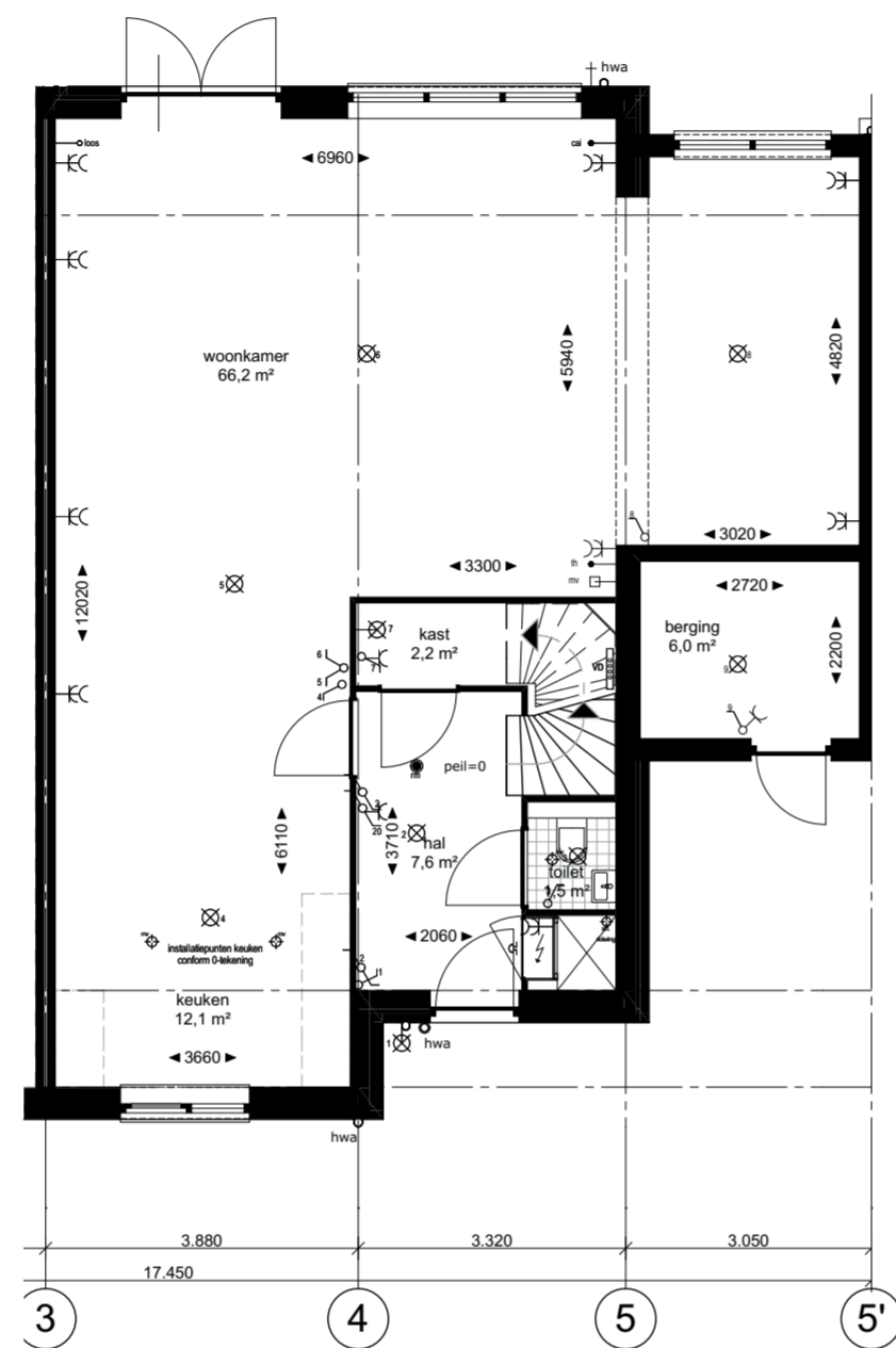
Begane grond 1:100
