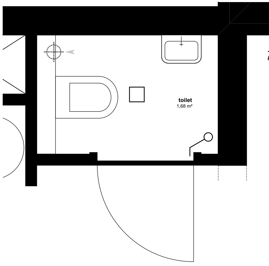
Toilet (1:20)
