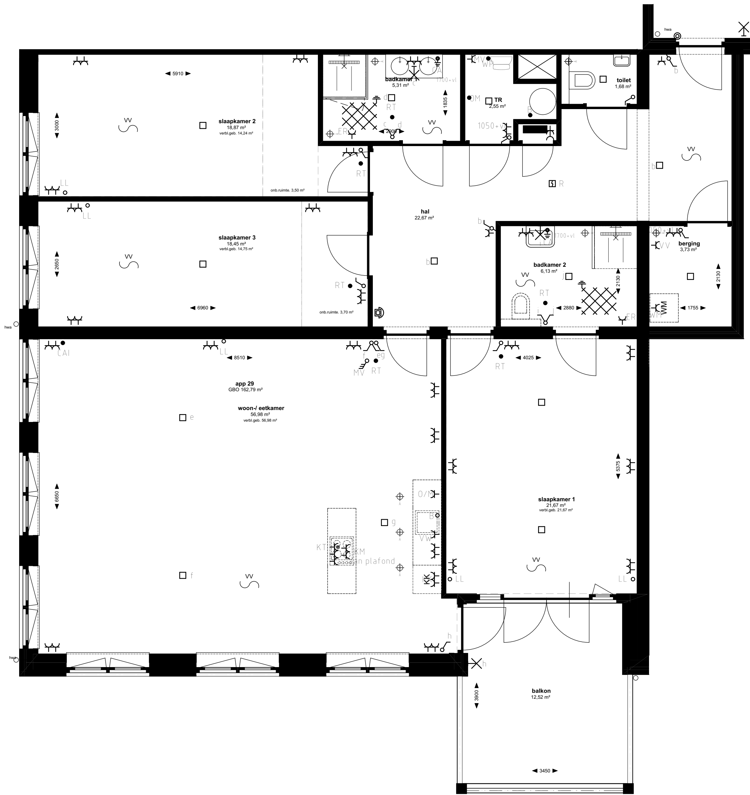
Appartement 29 (1:50)
