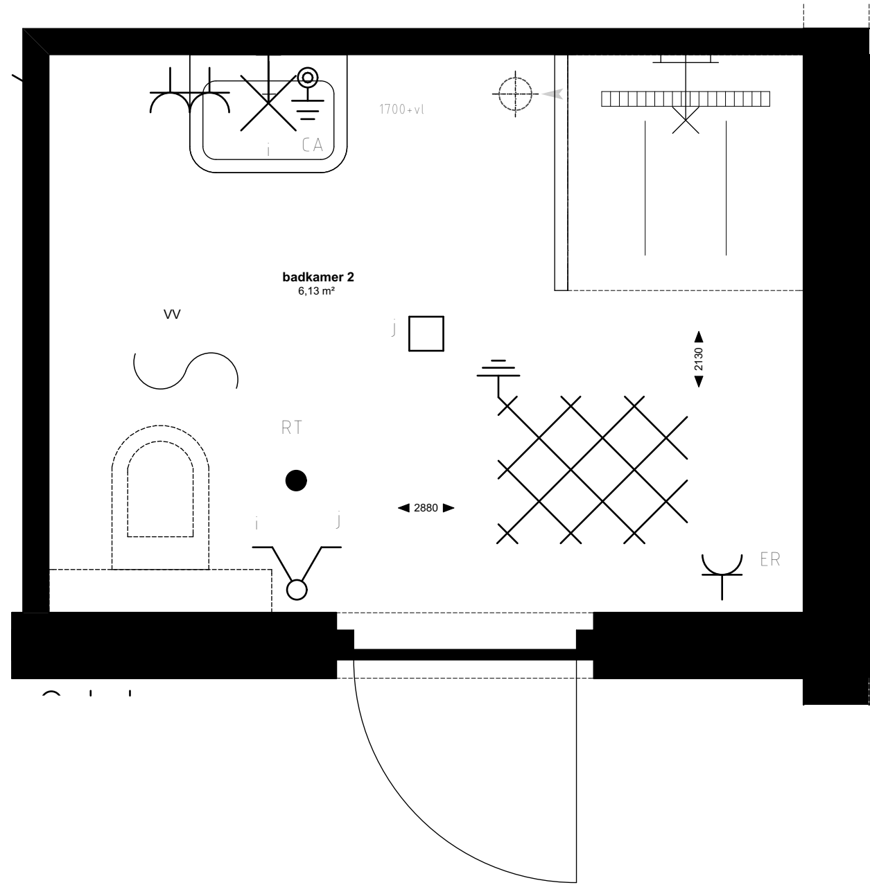
Badkamer 2 (1:20)
