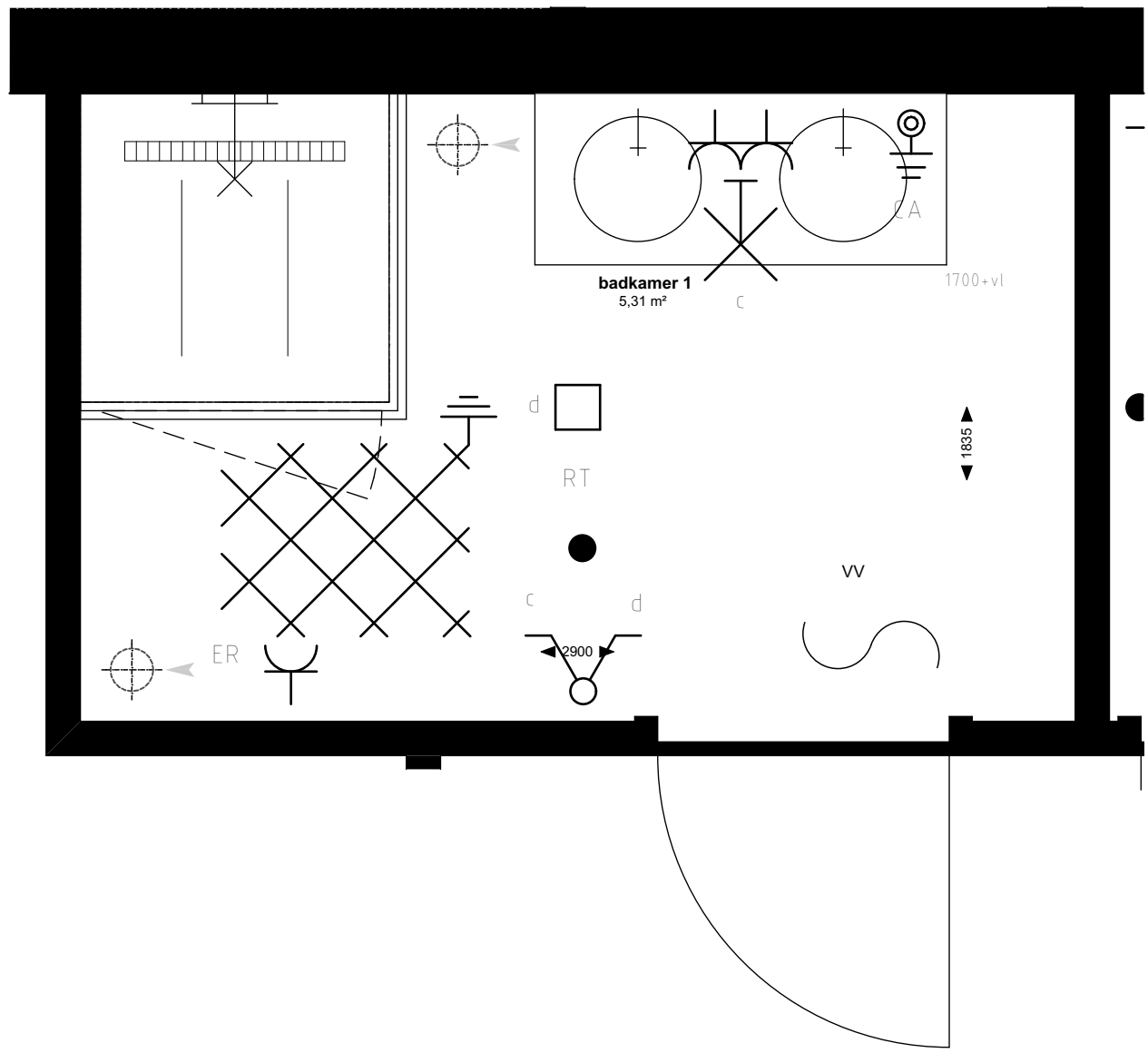
Badkamer 1 (1:20)
