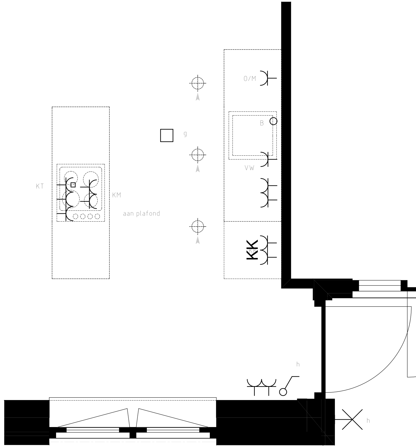
Keuken (1:20)
