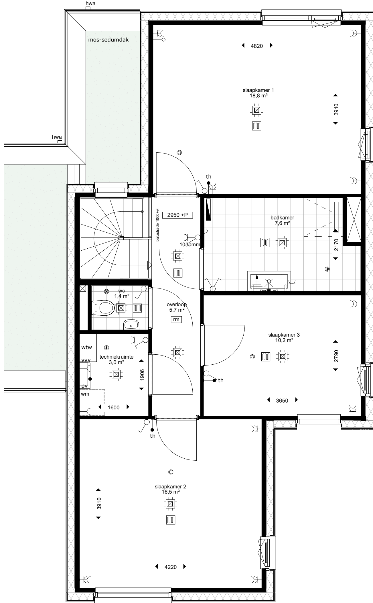
Eerste verdieping BNR 17 Geschakelde Watervilla L
