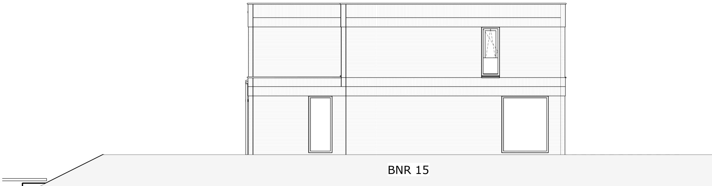
Rechter zijgevel
