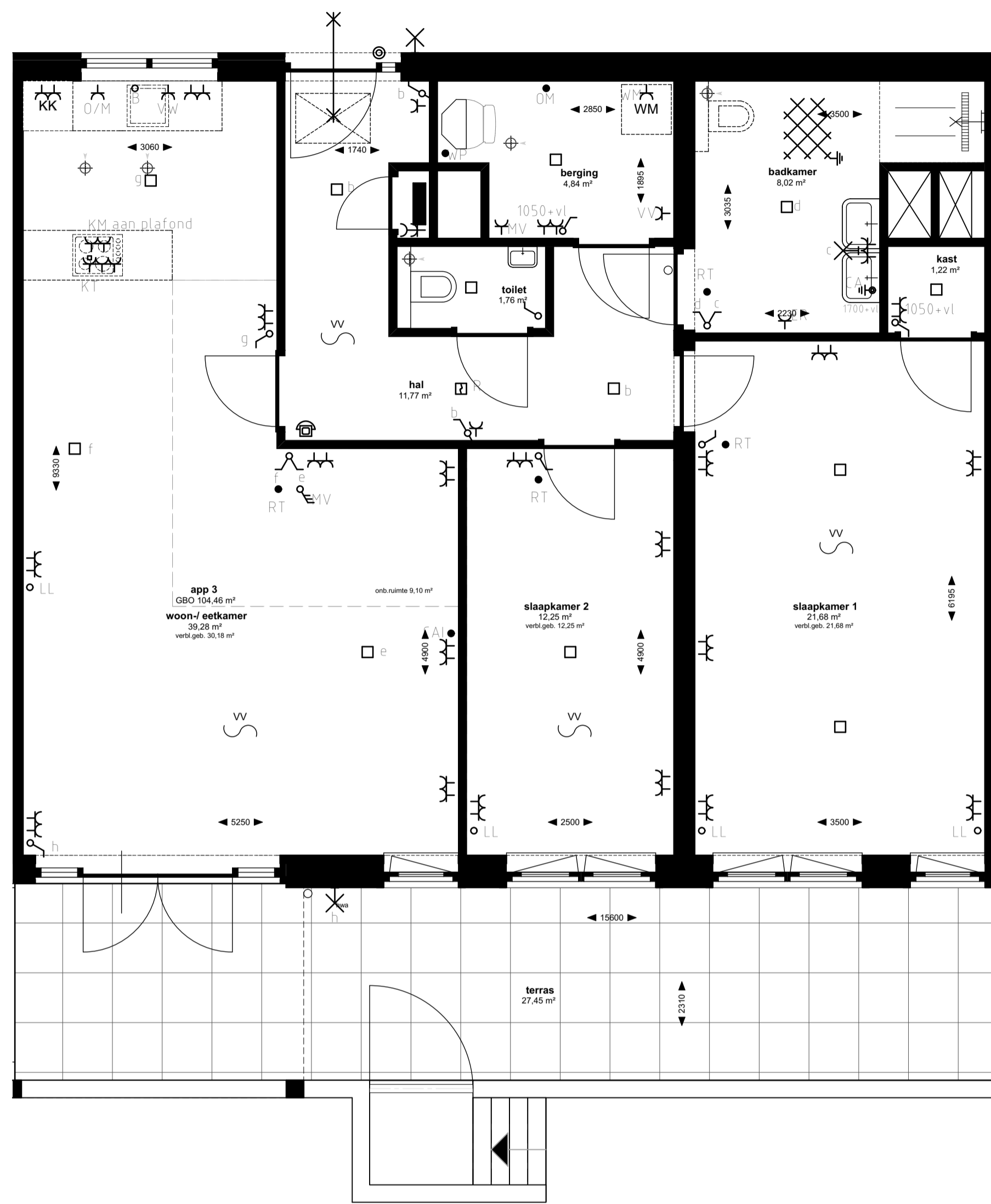
Appartement 3 (1:50)
