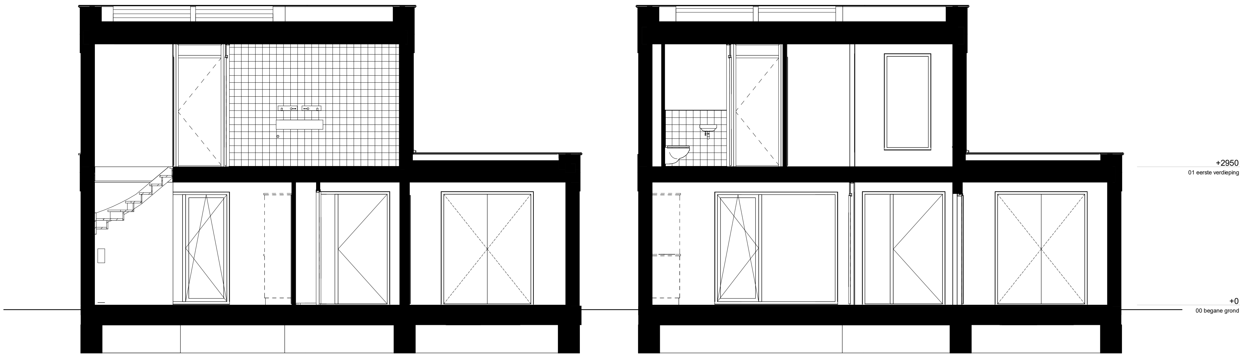
Doorsnede A
