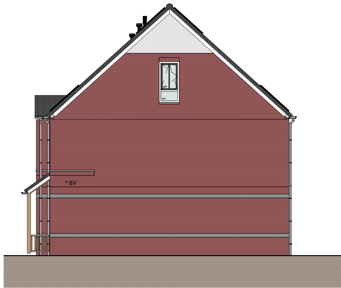
Rechterzij aanzicht (1:100)
