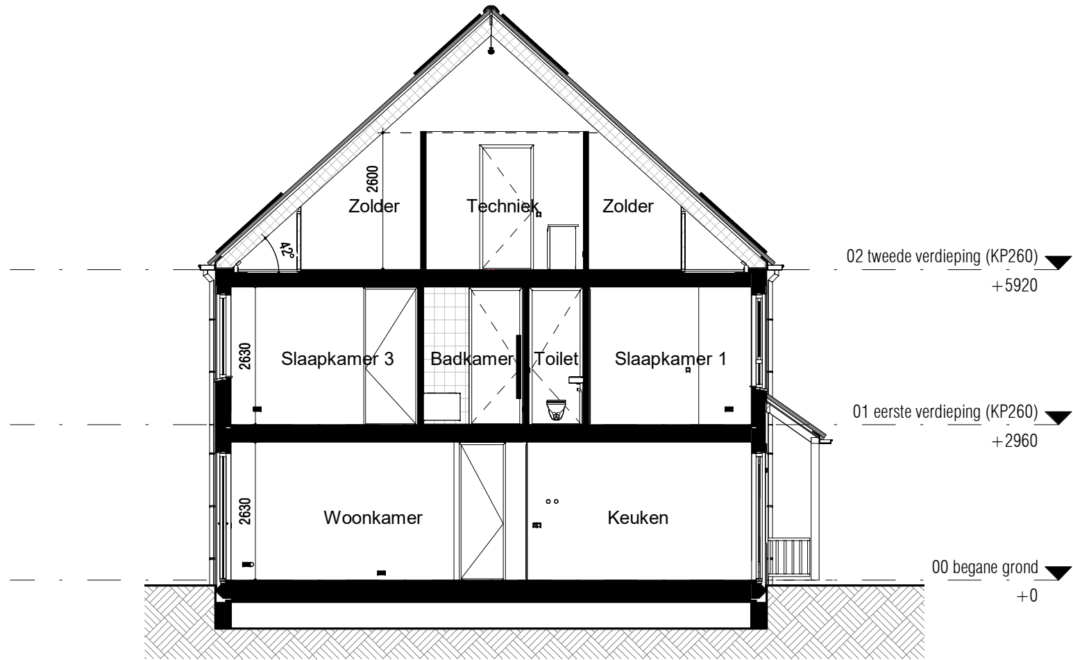
Doorsnede (1:100)
