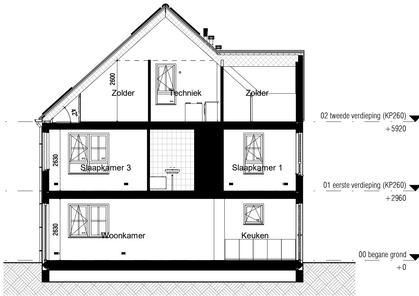
Doorsnede (1:100)
