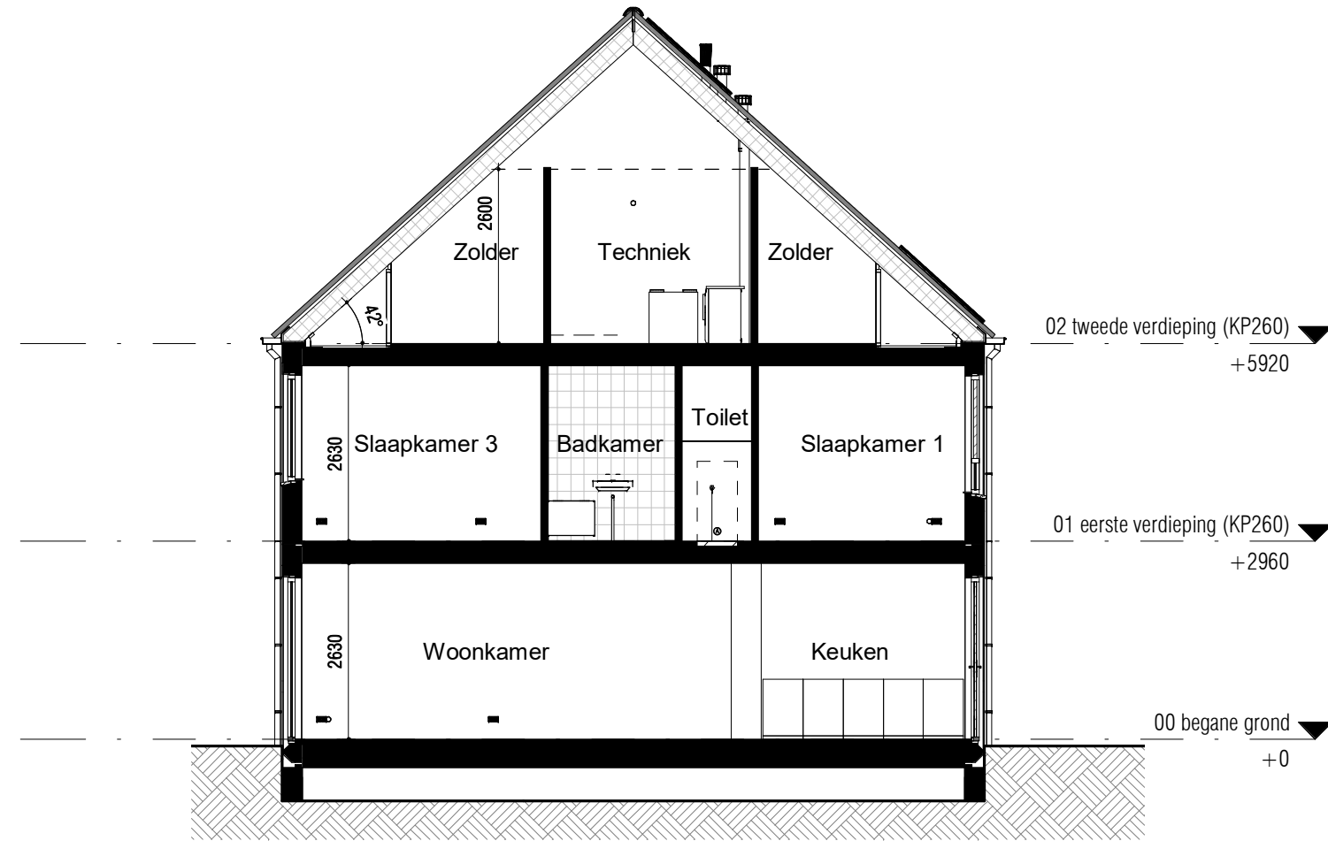
Doorsnede (1:100)
