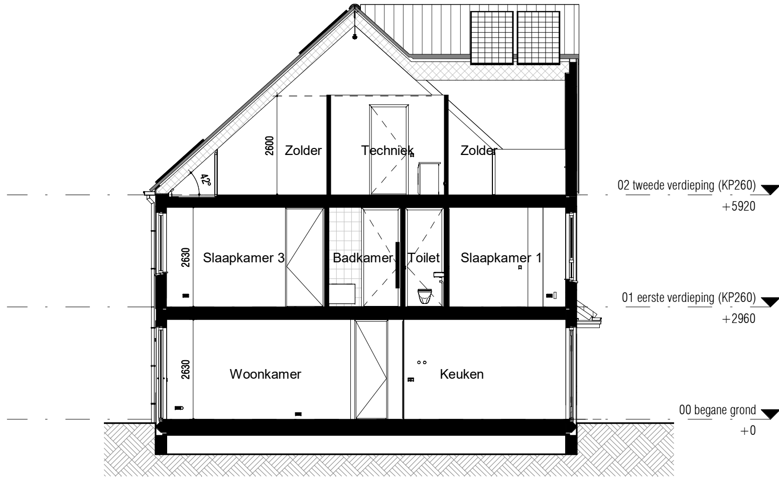
Doorsnede (1:100)
