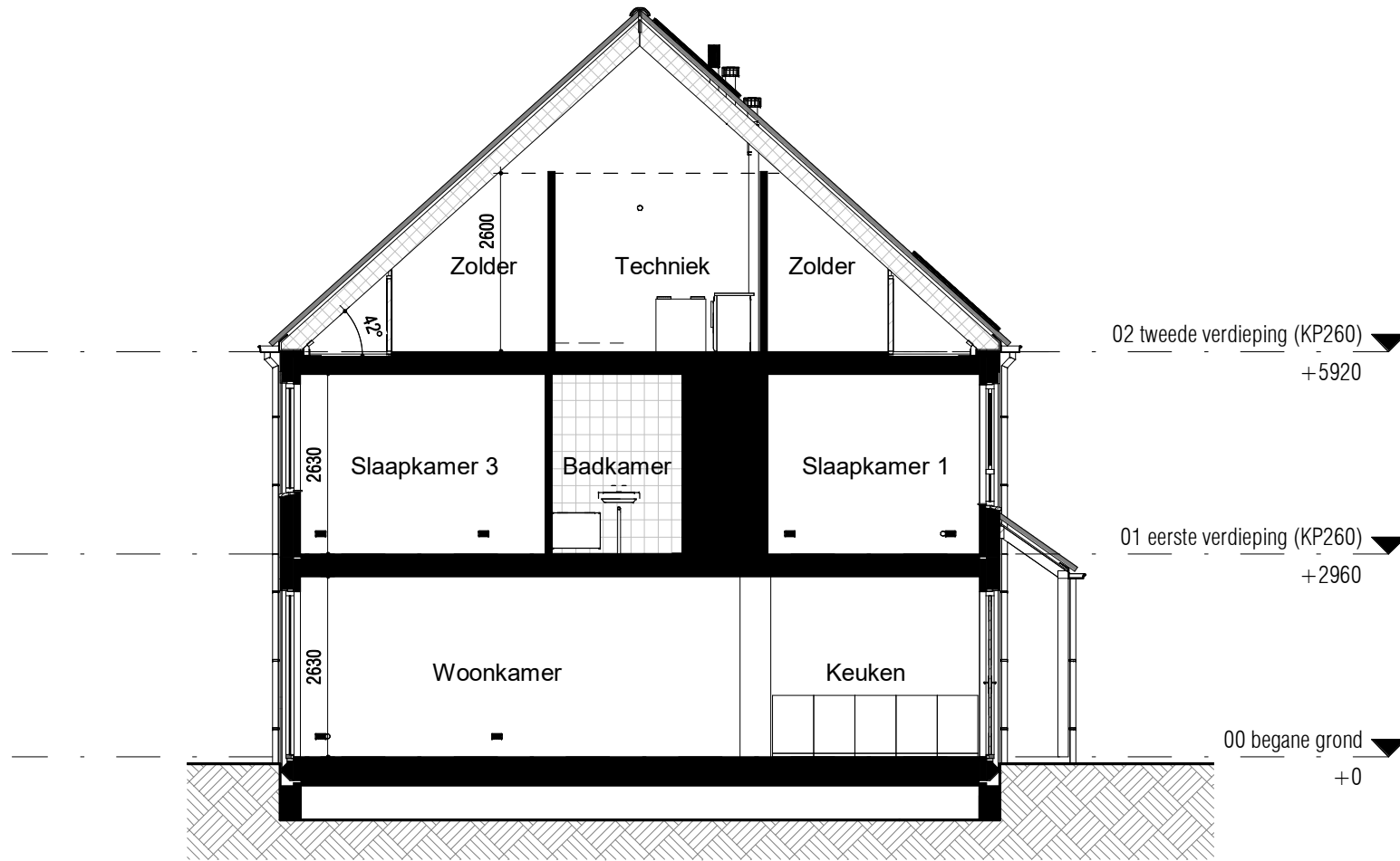
Doorsnede (1:100)
