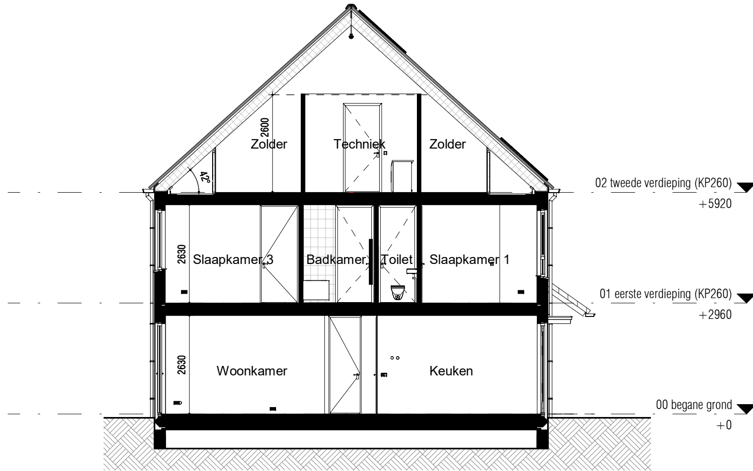
Doorsnede (1:100)
