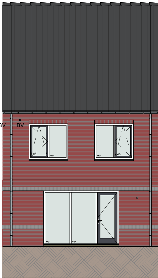
Achteraanzicht (1:100)
