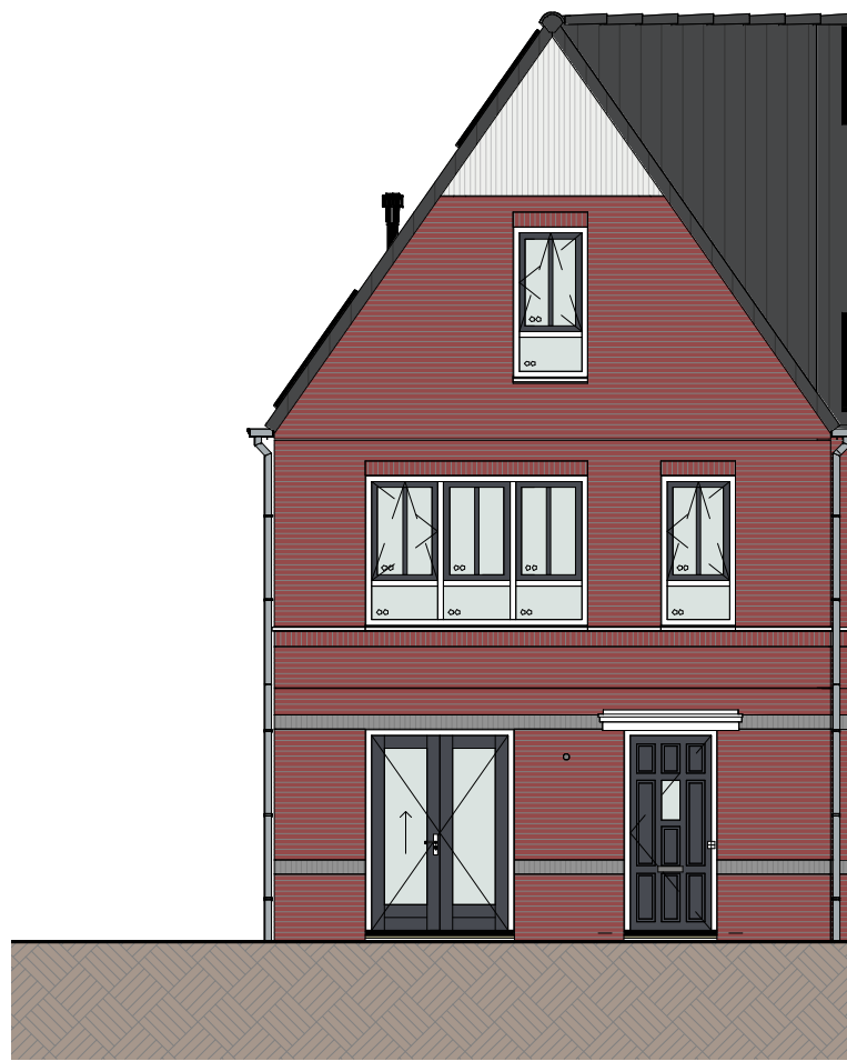
Vooraanzicht (1:100)
