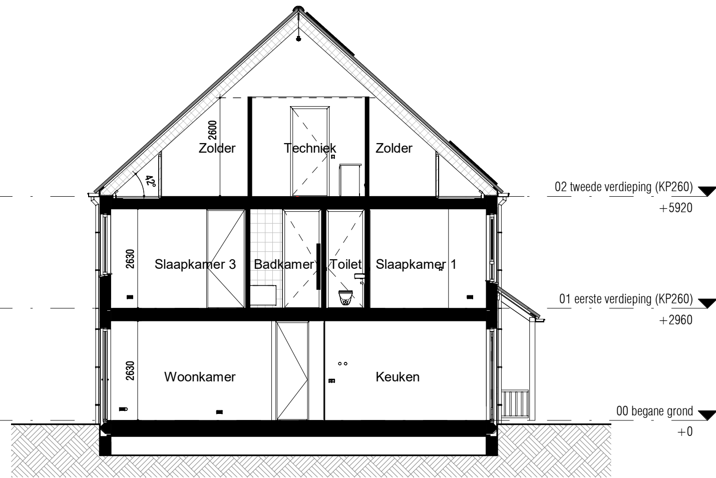
Doorsnede (1:100)
