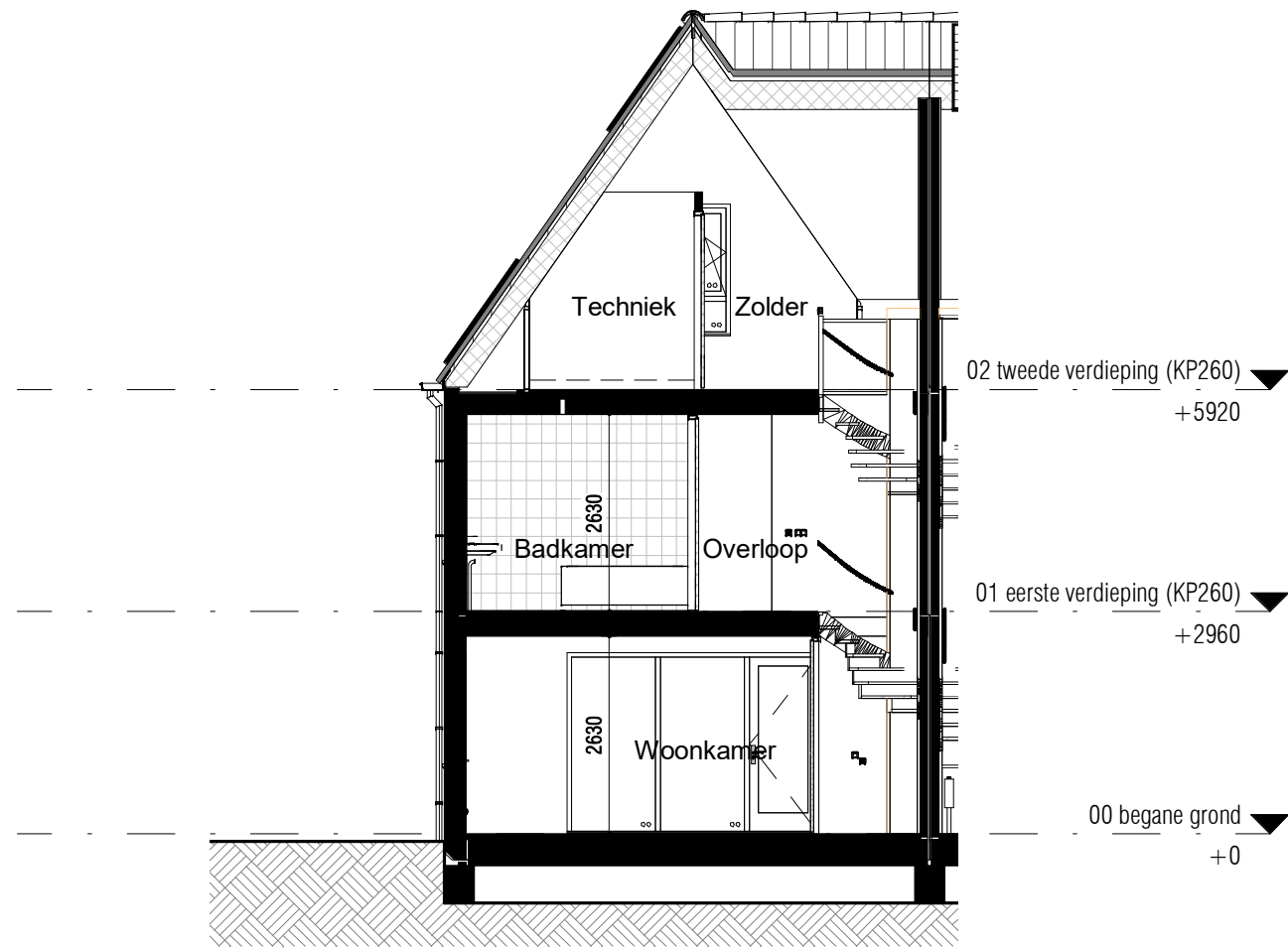
Doorsnede (1:100)
