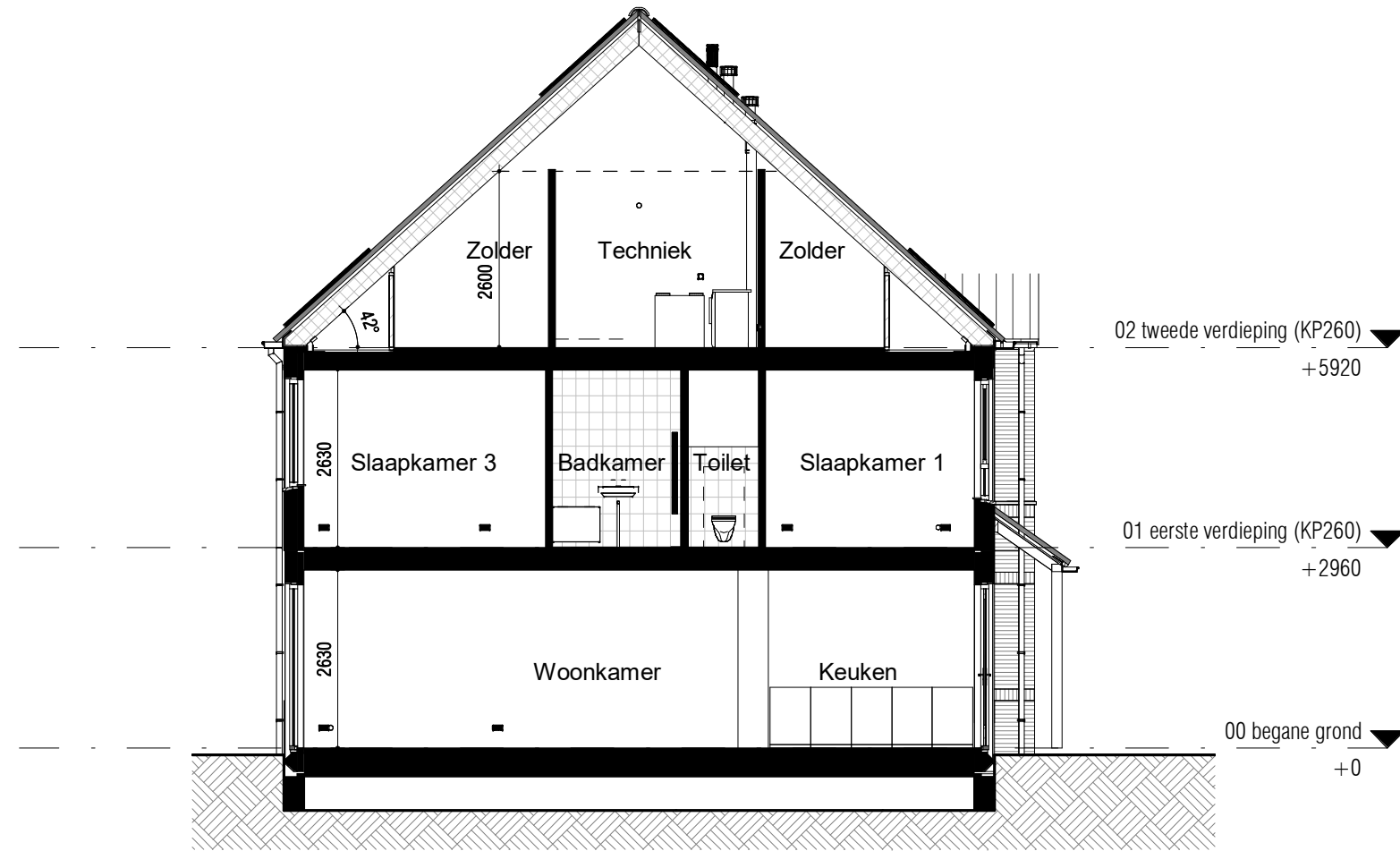
Doorsnede (1:100)
