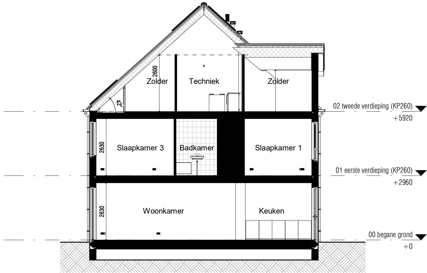
Doorsnede (1:100)
