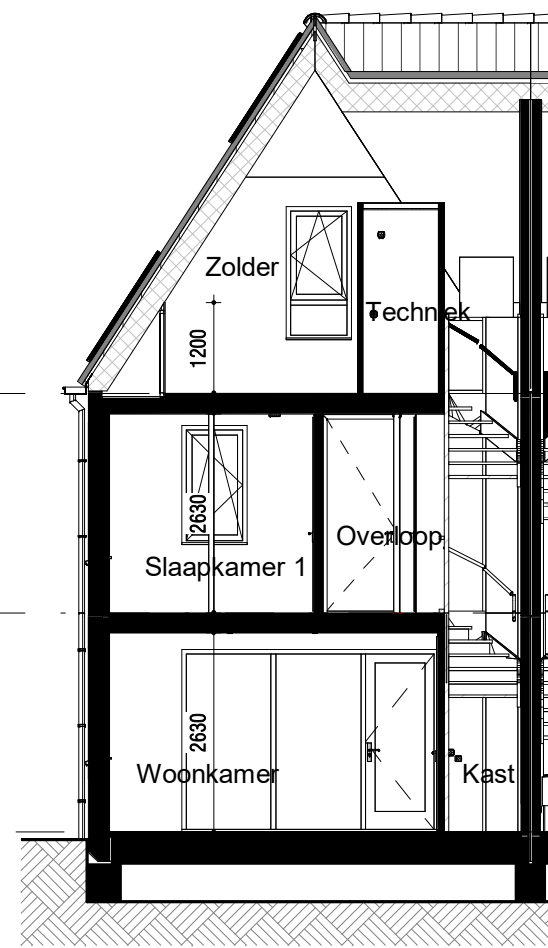
Doorsnede (1:100)
