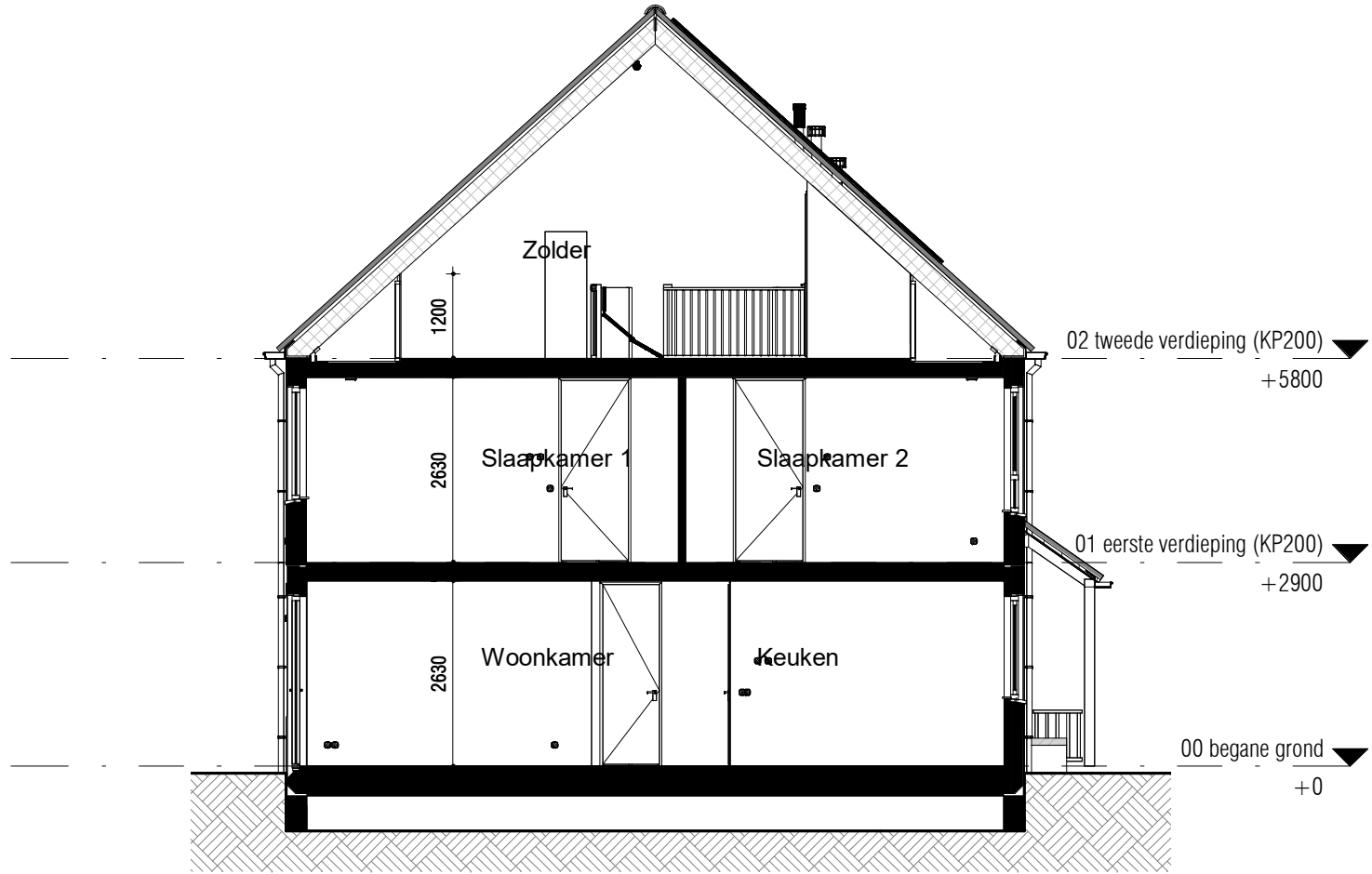
Doorsnede (1:100)
