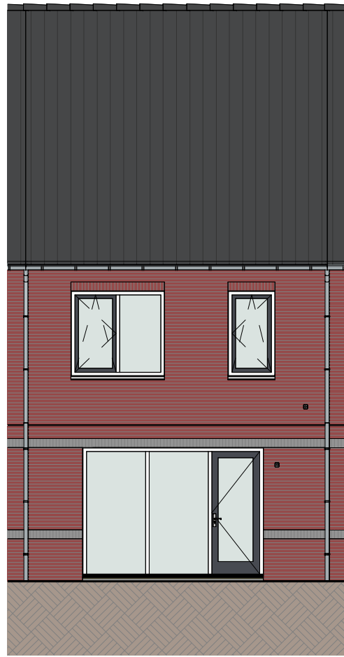
Achteraanzicht (1:100)
