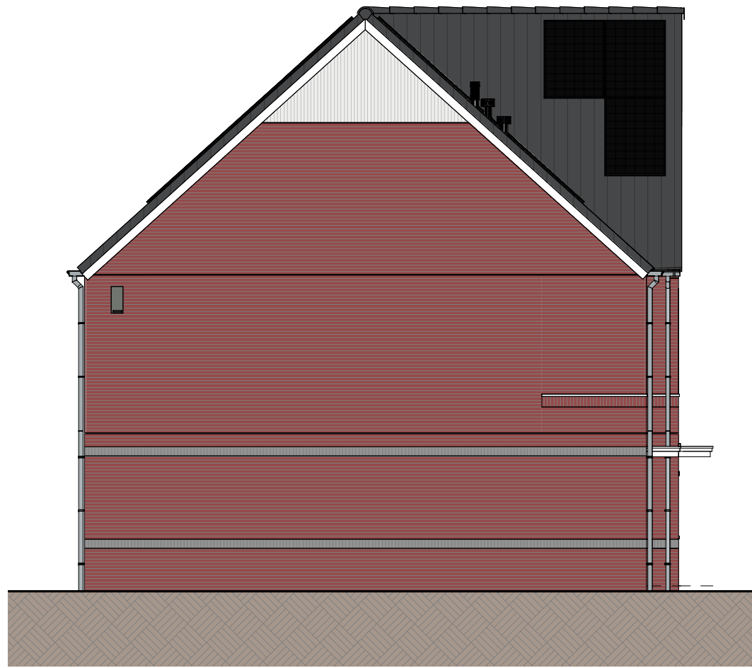
Linkerzijaanzicht (1:100)
