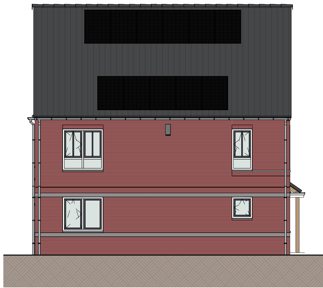
Linkerzijaanzicht (1:100)
