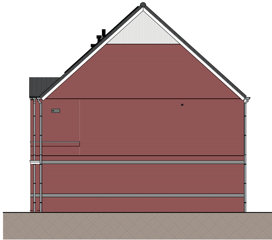
Rechterzij aanzicht (1:100)
