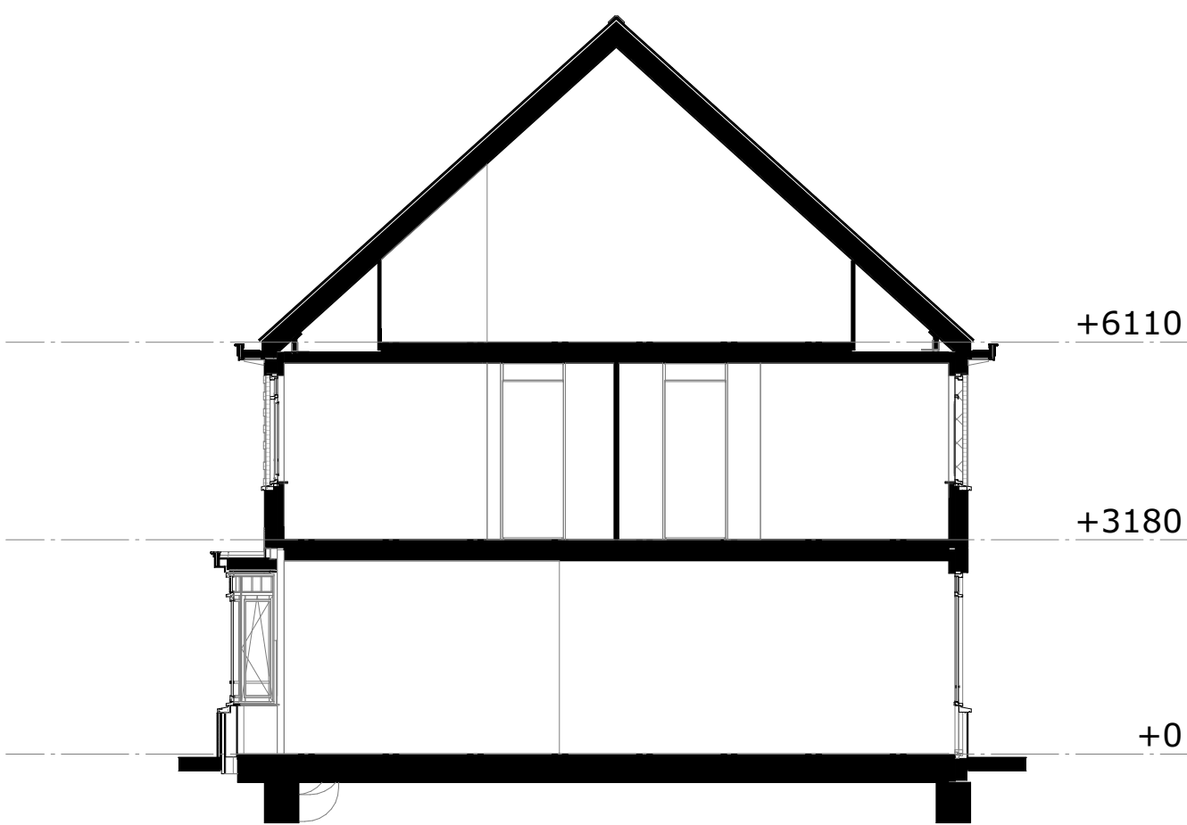
doorsnede A
