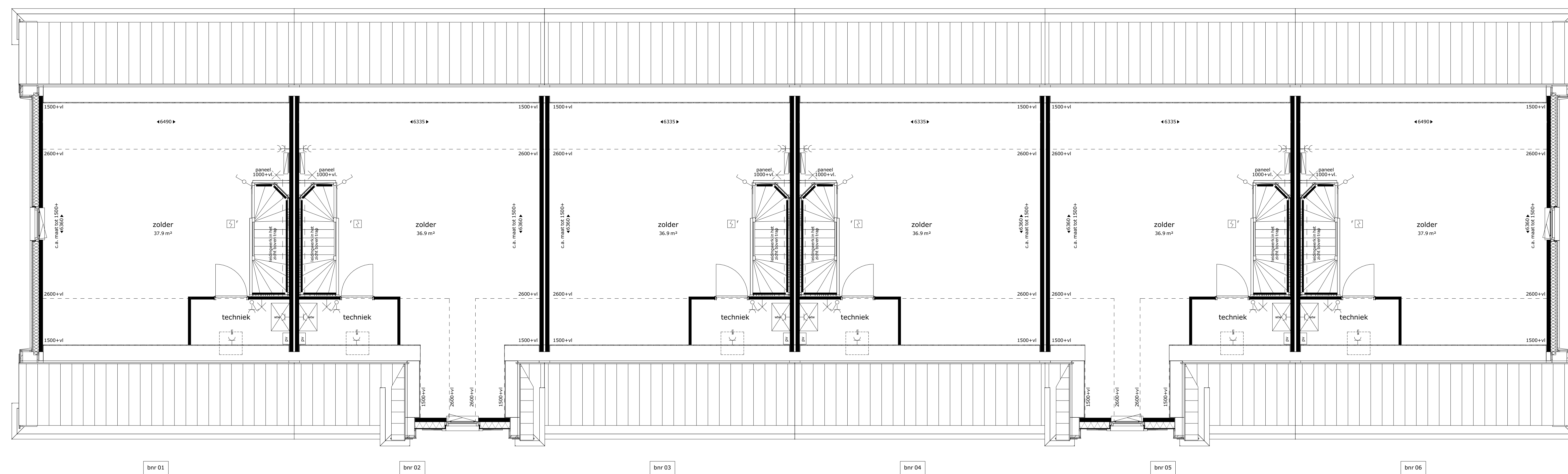
tweede verdieping
