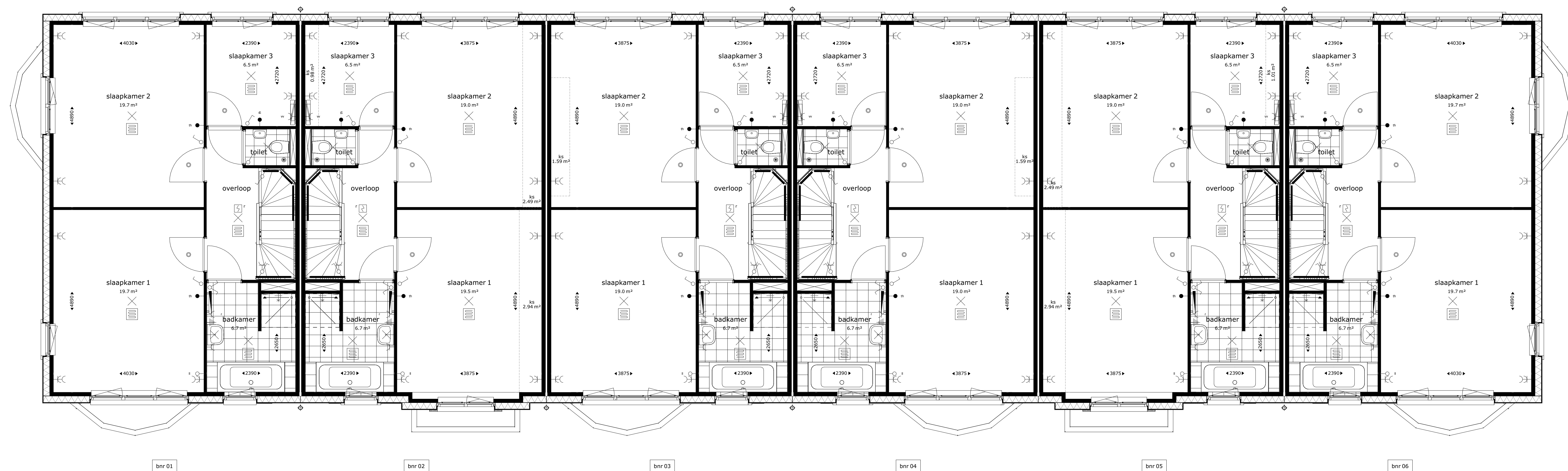
eerste verdieping
